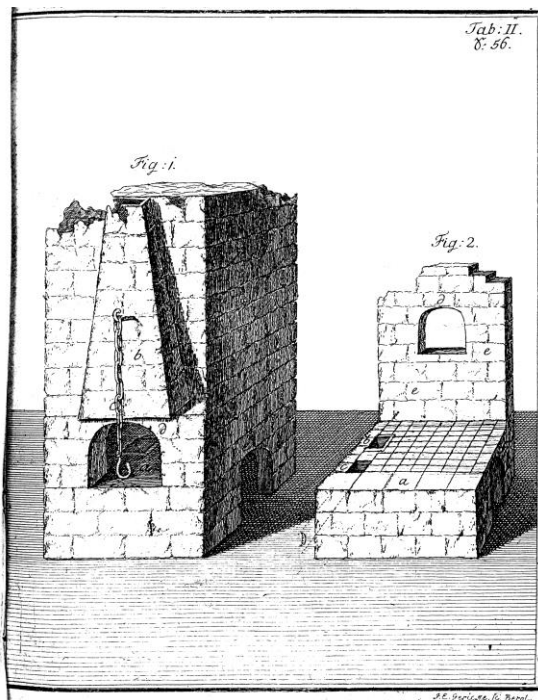
Fig. 8.12 - Fornace per calcinare il minerale: visione esterna e interna (con l'apertura che immette al condotto per il recupero dell'arsenico), dalla seconda parte della Cadmiologia di Johann Gottlob Lehmann (LEHMANN 1764, tav. II).
