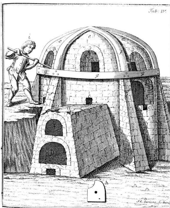
Fig. 8.13 - Fornace per la produzione dello smalto, dalla seconda parte della Cadmiologia di Johann Gottlob Lehmann (LEHMANN 1764, tav. IV).
