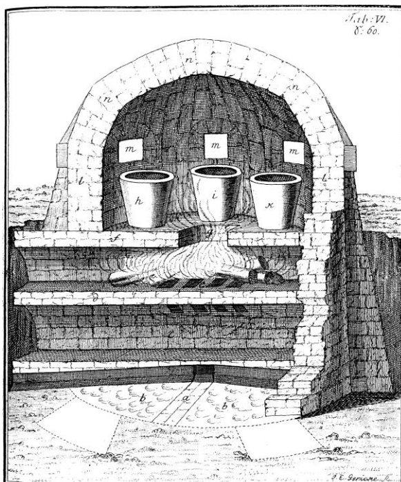
Fig. 8.14 - Sezione trasversale di fornace per la produzione dello smalto, dalla seconda parte della Cadmiologia di Johann Gottlob Lehmann (LEHMANN 1764, tav. VI).
