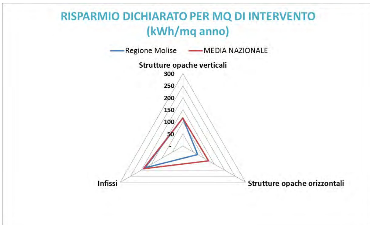
FIG. 16: RISPARMIO PER MQ DI INTERVENTO EFFETTUATO SULL'INVOLUCRO EDILIZIO IN RAPPORTO ALLA MEDIA NAZIONALE VALORI ESPRESI IN kWh/mq anno – REGIONE MOLISE, ANNO 2012
