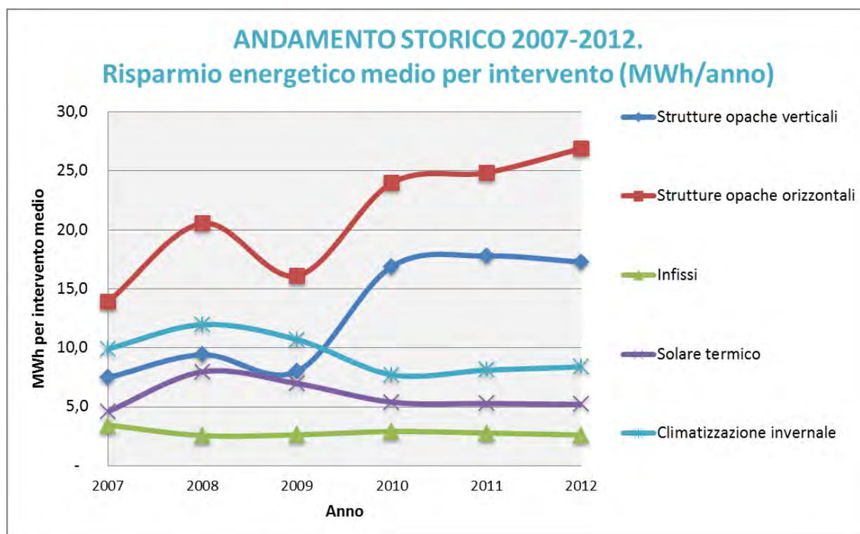
FIG.8.7 ANDAMENTO DEL VALORE DI RISPARMIO ENERGETICO MEDIO PER TIPOLOGIA DI INTERVENTO EFFETTUATO NEL PERIODO 2007-2012. VALORI ESPRESI IN MWh/ANNO
