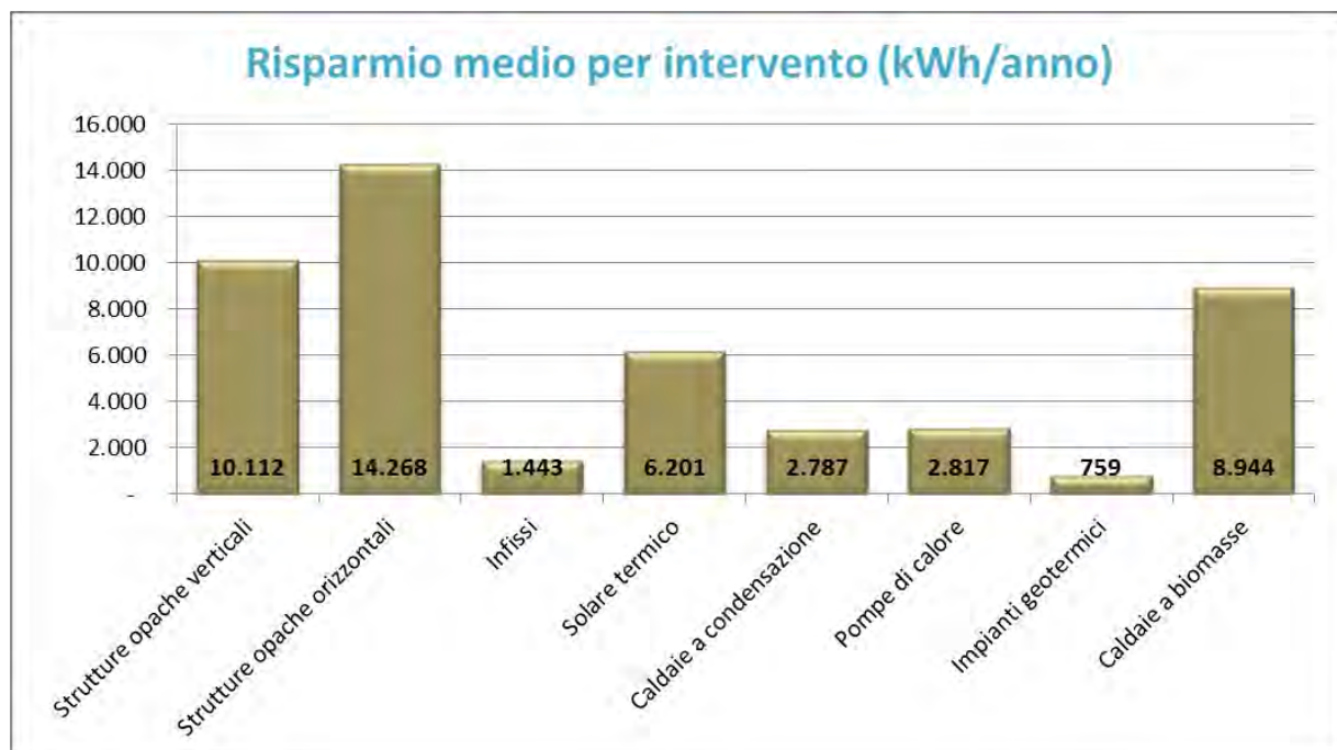
FIG. 9: RISPARMIO MEDIO ANNUO ASSOCIATO ALLA SINGOLA TIPOLOGIA DI INTERVENTO. VALORI ESPRESSI IN kWh/ANNO – REGIONE SARDEGNA, ANNO 2012
