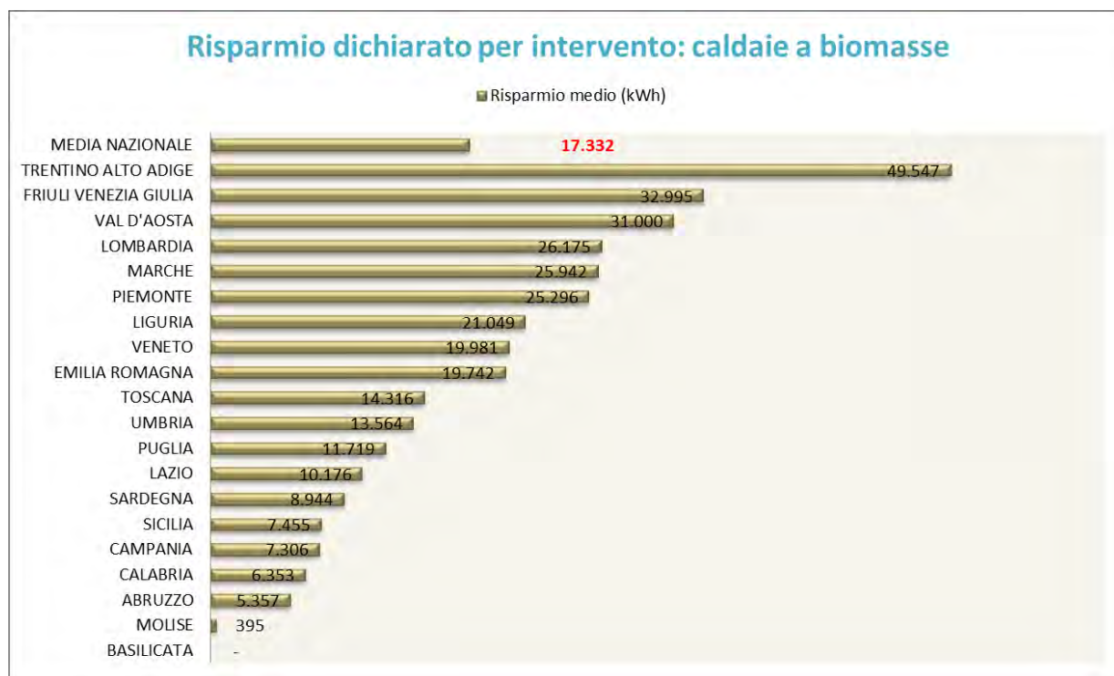
FIGURA 3.2 SOSTITUZIONE DI IMPIANTI TERMICI CON CALDAIE A BIOMASSE. RISPARMIO REALIZZATO CON L'INTERVENTO MEDIO EFFETTUATO NEL 2012 (KWh/ANNO)
