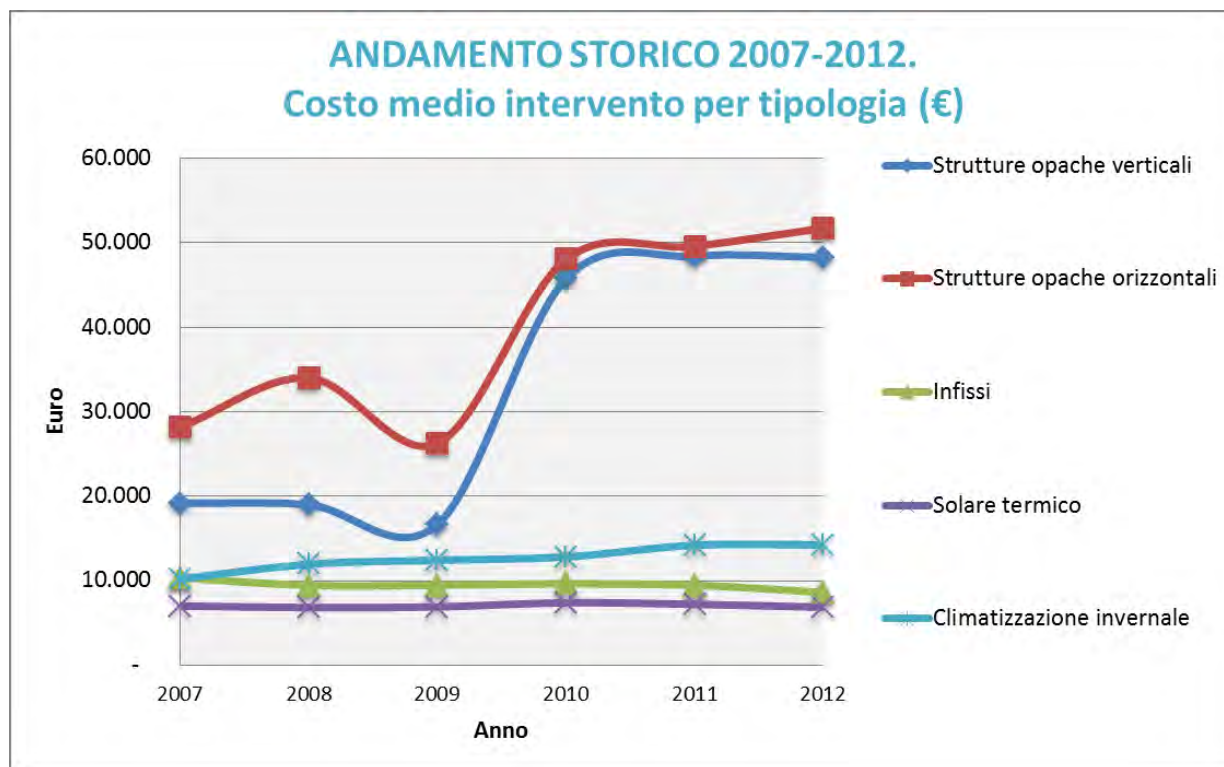
FIG.8.6 ANDAMENTO DEL VALORE DI COSTO MEDIO PER TIPOLOGIA DI INTERVENTO EFFETTUATO NEL PERIODO 2007-2012. VALORI ESPRESI IN €
