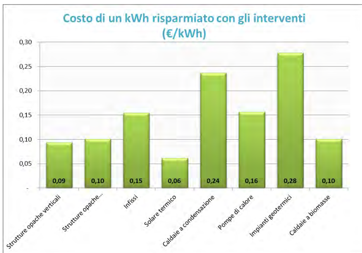
FIG. 10: COSTO DI UN kWh ANNO RISPARMIATO ASSOCIATO ALLE DIVERSE TIPOLOGIE DI INTERVENTO VALORI ESPRESI IN €/kWh – REGIONE UMBRIA, ANNO 2012
