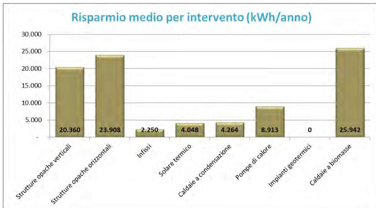
FIG. 9: RISPARMIO MEDIO ANNUO ASSOCIATO ALLA SINGOLA TIPOLOGIA DI INTERVENTO. VALORI ESPRESSI IN kWh/ANNO – REGIONE MARCHE, ANNO 2012
