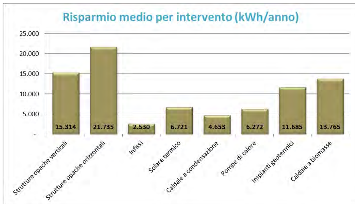
FIG. 9: RISPARMIO MEDIO ANNUO ASSOCIATO ALLA SINGOLA TIPOLOGIA DI INTERVENTO. VALORI ESPRESI IN kWh/ANNO – PROVINCIA AUTONOMA DI TRENTO, ANNO 2012
