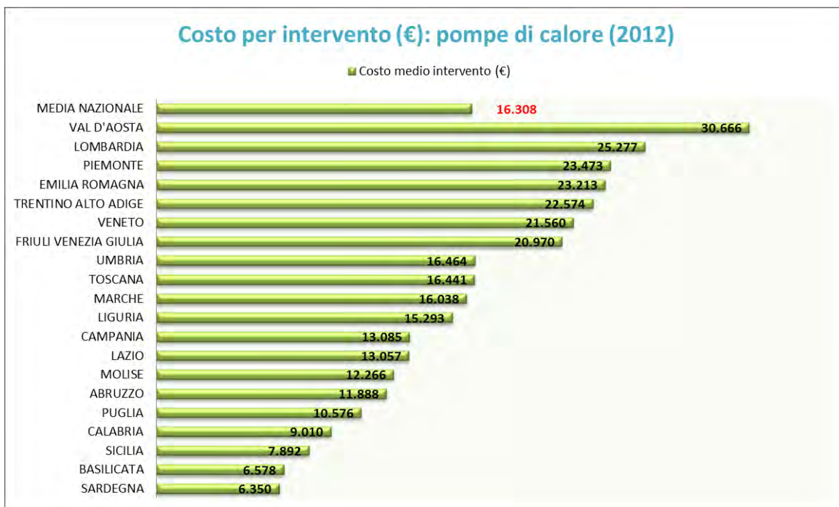
FIG.6.17 POMPE DI CALORE. COSTO MEDIO DELL'INTERVENTO. I VALORI NUMERICI SONO RIFERITI AL VALORE COMPLESSIVO DI PRATICHE INVIATE NEL 2010
