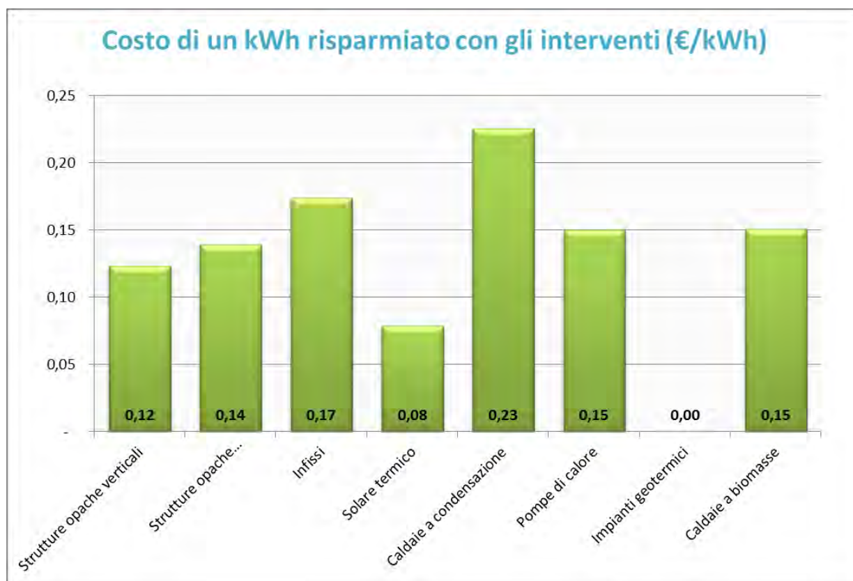
FIG. 10: COSTO DI UN kWh ANNO RISPARMIATO ASSOCIATO ALLE DIVERSE TIPOLOGIE DI INTERVENTO VALORI ESPRESSI IN €/kWh – REGIONE MARCHE, ANNO 2012
