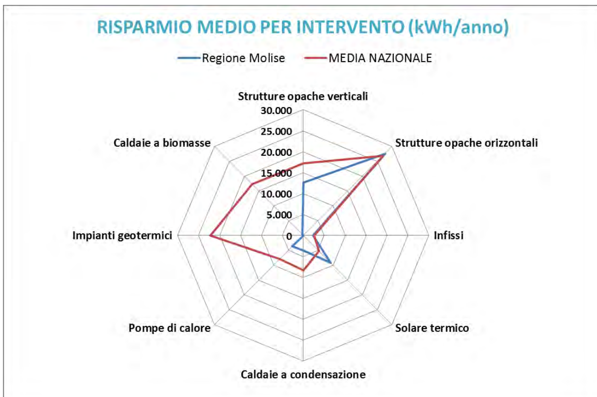
FIG. 15: RISPARMIO MEDIO ANNUO PER TIPOLOGIA DI INTERVENTO IN RAPPORTO ALLA MEDIA NAZIONALE VALORI ESPRESI IN kWh/ANNO – REGIONE MOLISE, ANNO 2012
