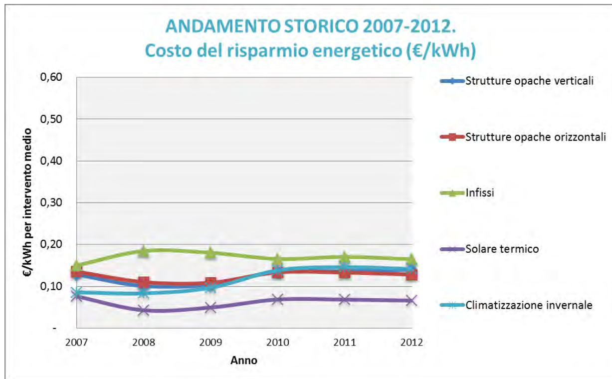
FIG.8.8 ANDAMENTO DEL VALORE DI COSTO MEDIO PER TIPOLOGIA DI INTERVENTO EFFETTUATO NEL PERIODO 2007-2012. VALORI ESPRESSI IN €/kWh
