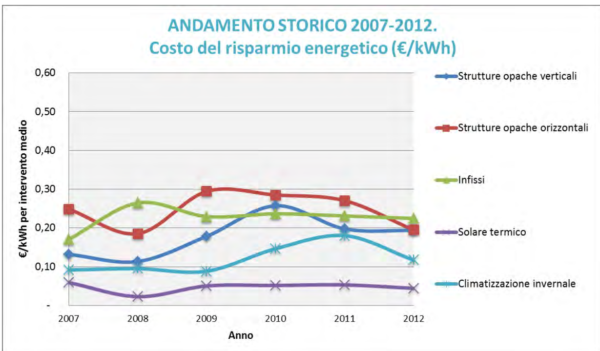
FIG. 18: REGIONE LAZIO DATI STORICI ANNI 2007-2012: ANDAMENTO DEL COSTO DEL RISPARMIO ENERGETICO UNITARIO DISTINTO PER TIPOLOGIA DI INTERVENTO. VALORI ESPRESSE IN €/kWh
