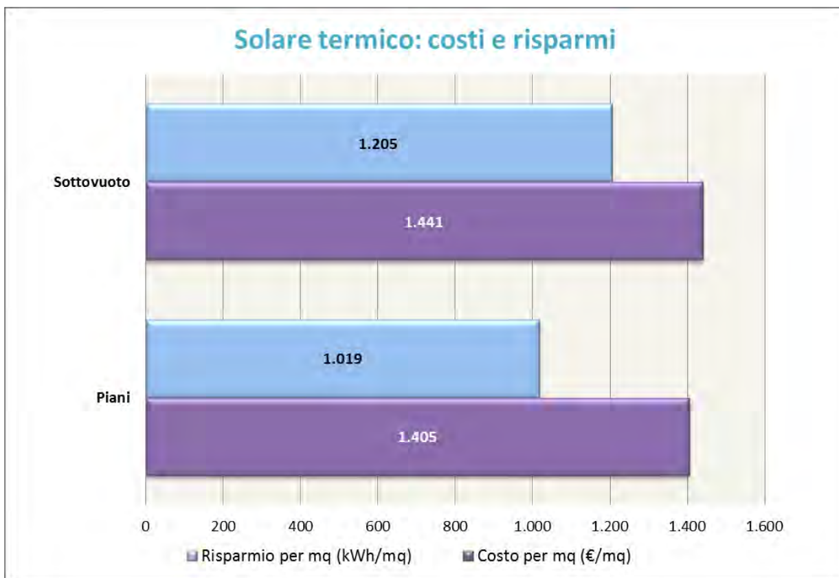
FIG.5.11 COSTO MEDIO DEI PANNELLI IN RELAZIONE AI RISPARI MEDI OTTENUTI PER TIPOLOGIA.
