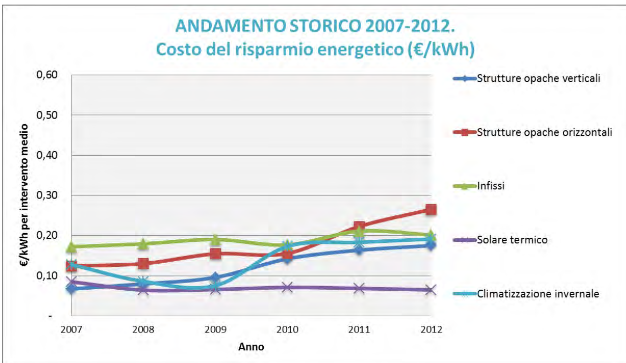
FIG. 18: REGIONE TRENTINO-ALTO ADIGE DATI STORICI ANNI 2007-2012: ANDAMENTO DEL COSTO DEL RISPARMIO ENERGETICO UNITARIO DISTINTO PER TIPOLOGIA DI INTERVENTO. VALORI ESPRESI IN €/kWh
