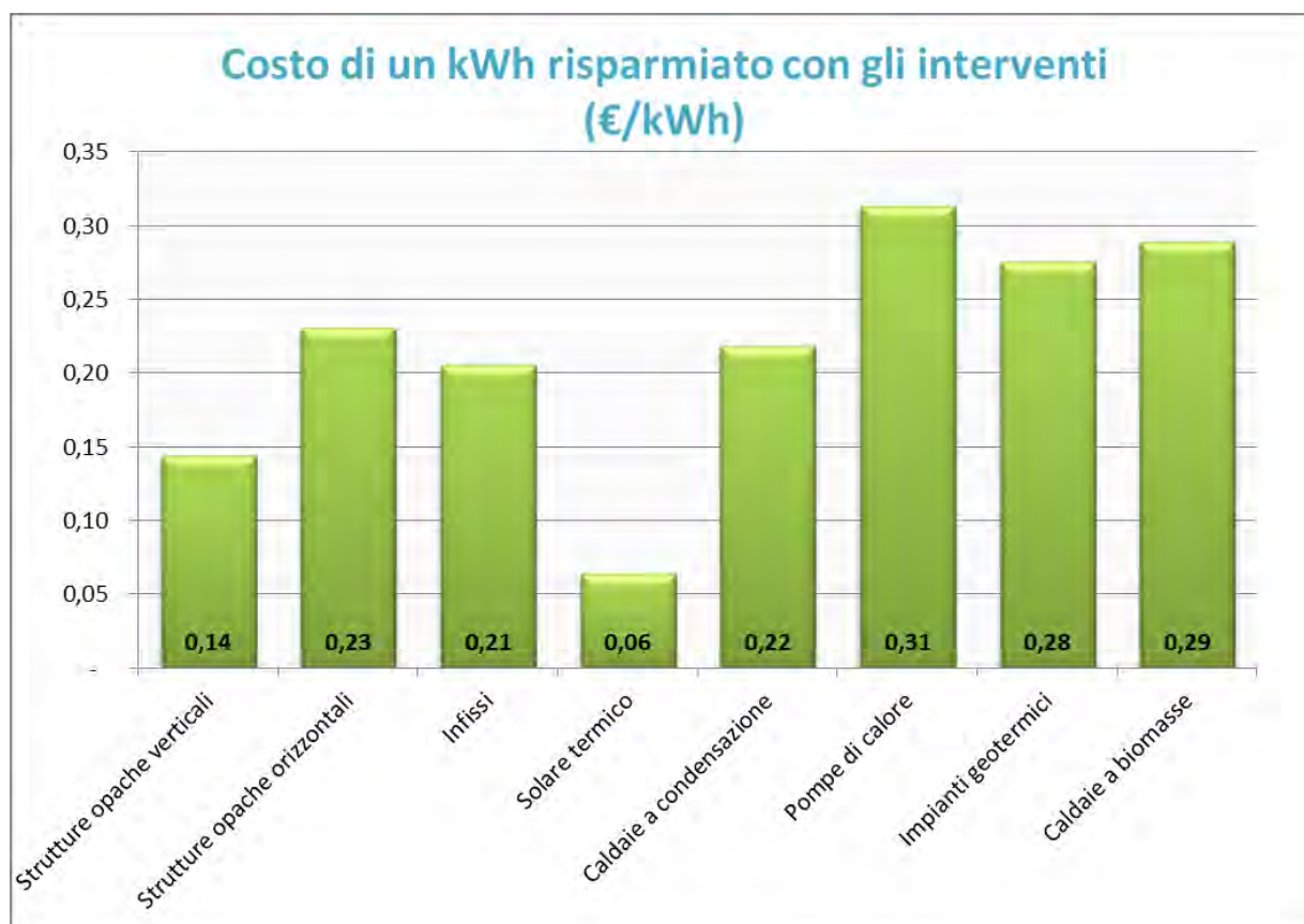
FIG. 10: COSTO DI UN kWh ANNO RISPARMIATO ASSOCIATO ALLE DIVERSE TIPOLOGIE DI INTERVENTO VALORI ESPRESI IN €/kWh – PROVINCIA AUTONOMA DI TRENTO, ANNO 2012
