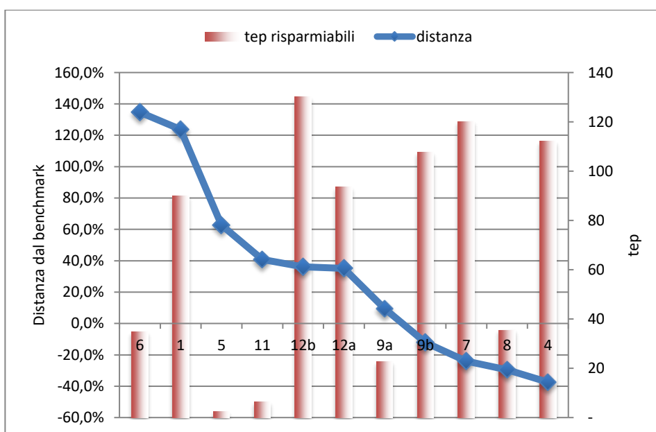
Fig. 8 – Distanza dal benchmark e tep risparmiabili
