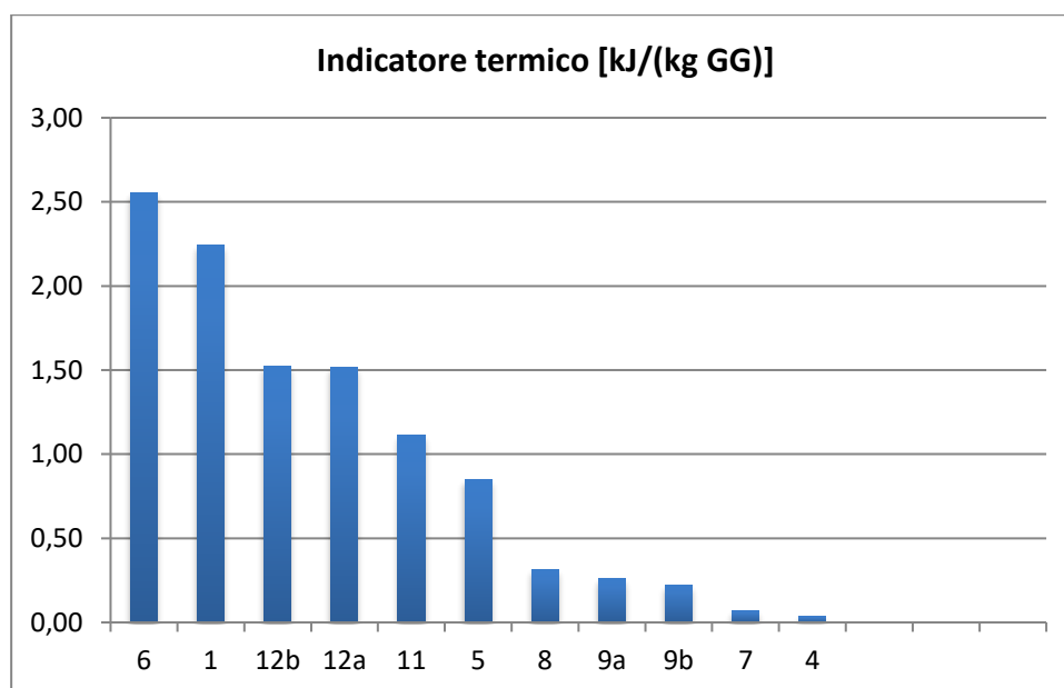
Fig. 3a – IPE termico per grado giorno
