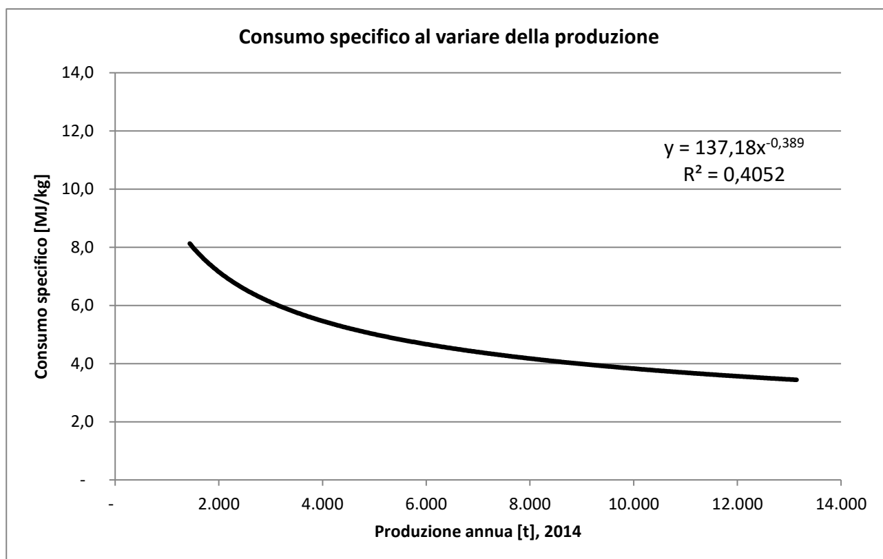
Fig. 6 – Consumo specifico Vs produzione annua
