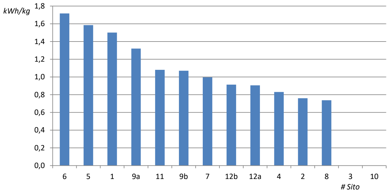
Fig. 2 – IPE elettrico
