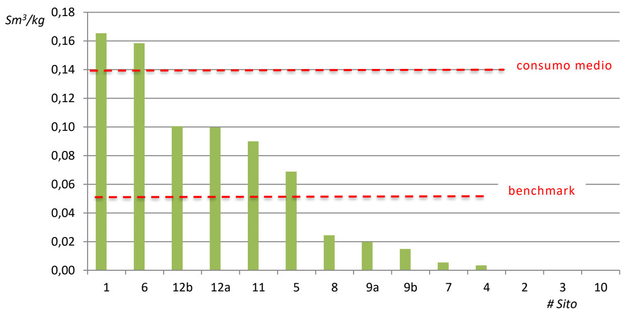
Fig. 5 – Confronto tra IPE termico e benchmark
