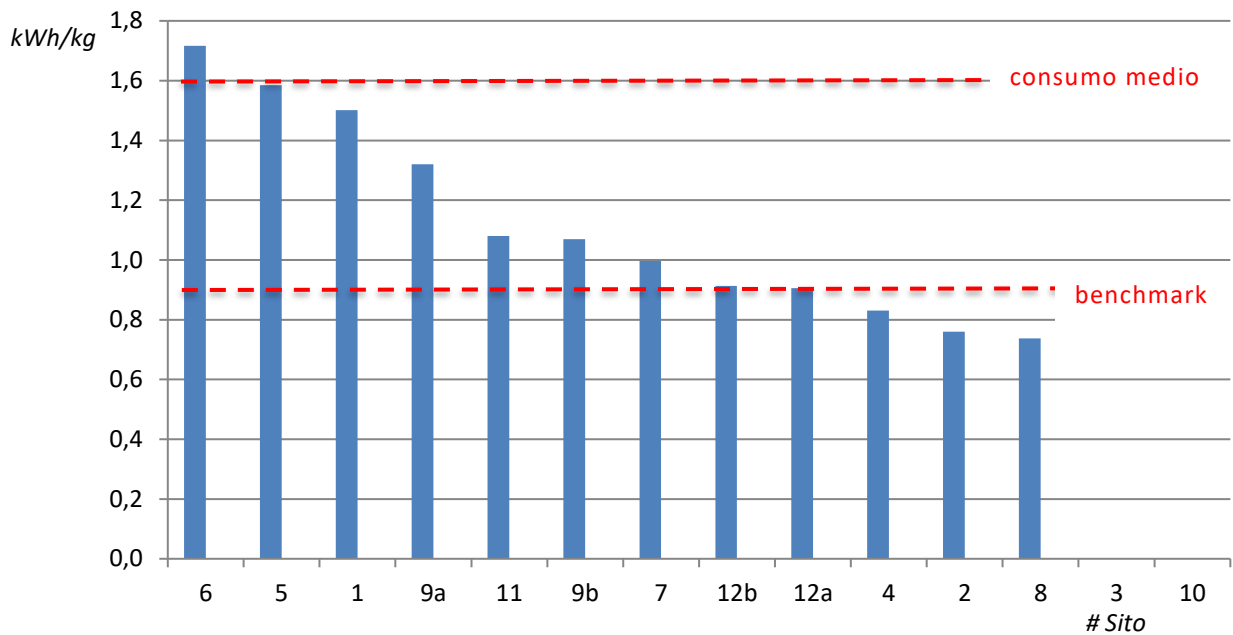
Fig. 4 – Confronto tra IPE elettrico e benchmark
