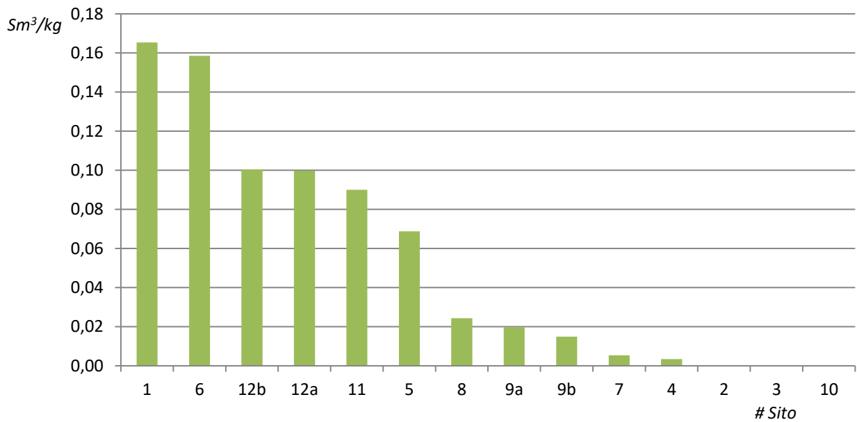
Fig. 3 – IPE termico
