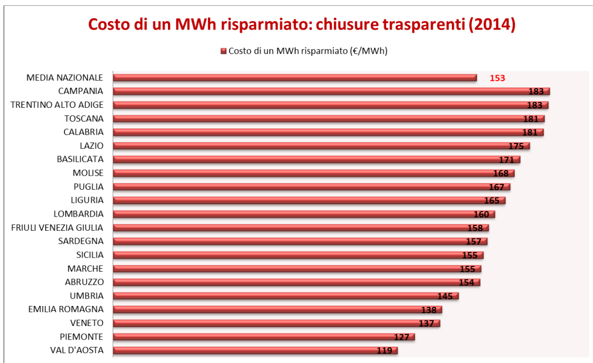
FIG.4.22 COSTO MEDIO ANNUO DI OGNI MWh RISPARMIATO PER LA SOSTITUZIONE DI INFISSI
