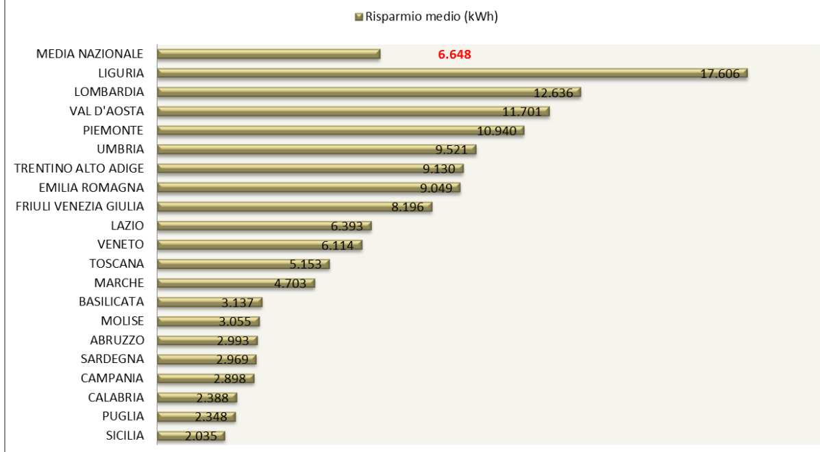
FIG.6.3 SOSTITUZIONE DI IMPIANTI TERMICI. RISPARMIO REALIZZATO CON L'INTERVENTO MEDIO. I VALORI NUMERICI SONO ESPRESSI IN kWh/ANNO E RIFERITI AL VALORE COMPLESSIVO DI PRATICHE INVIATE NEL 2014
