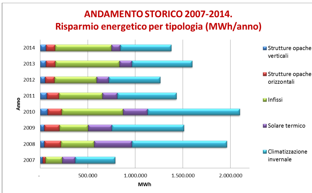
FIG.8.3 QUADRO DI SINTESI RELATIVO AL TOTALE DEI RISPARMI ENERGETICI ASSOCIATI ALLA CAMPAGNA DELLE DETRAZIONI FISCALI DEL 65% NEL 2014
