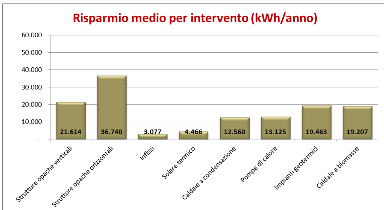
FIG. 10 RISPARMIO MEDIO ANNUO ASSOCIATO ALLA SINGOLA TIPOLOGIA DI INTERVENTO. VALORI ESPRESSI IN kWh/ANNO – REGIONE LOMBARDIA, ANNO 2014
