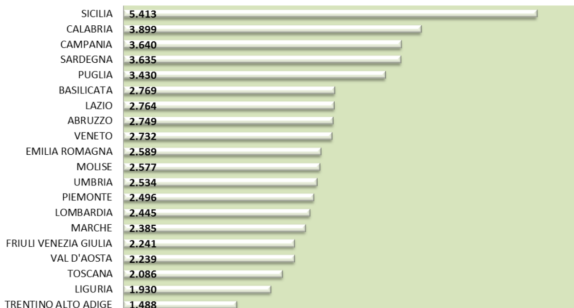
FIG.4.20 SOSTITUZIONE INFISSI. RISPARMIO REALIZZATO CON L'INTERVENTO MEDIO EFFETTUATO NEL 2014. DATO NORMALIZZATO IN FUNZIONE DEI GRADI GIORNO REGIONALI. (kWh/ANNO)
