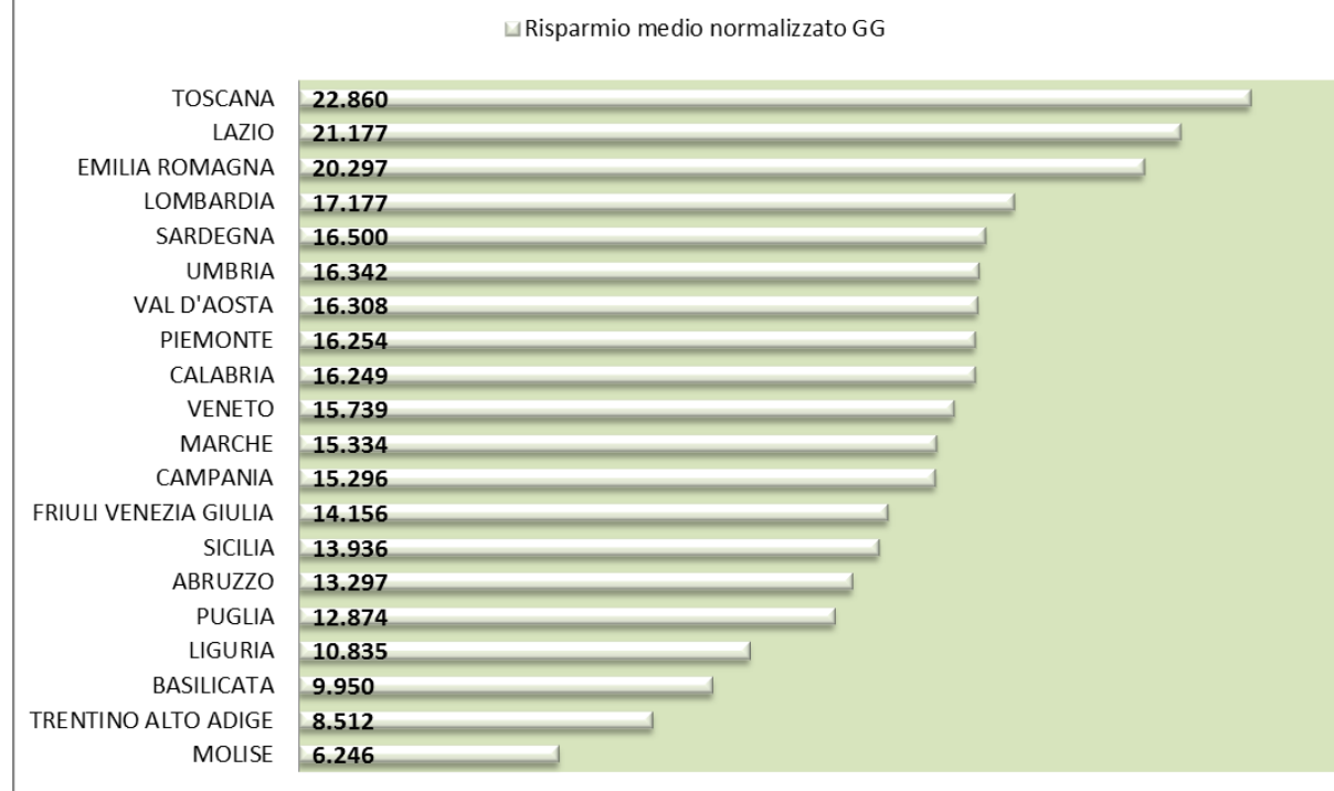
FIG.4.12 INTERVENTI SU STRUTTURE OPACHE VERTICALI. RISPARMIO REALIZZATO CON L'INTERVENTO MEDIO EFFETTUATO NEL 2014. DATO NORMALIZZATO IN FUNZIONE DEI GRADI GIORNO REGIONALI (kWh/ANNO)
