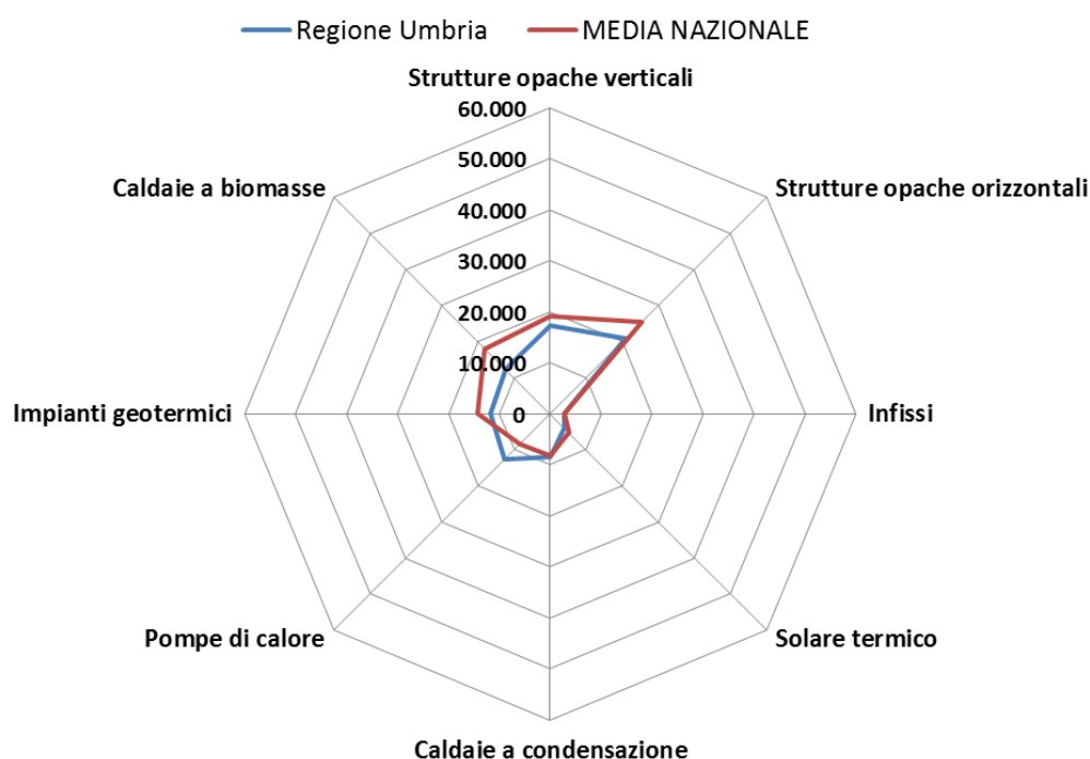
FIG. 15 RISPARMIO MEDIO ANNUO PER TIPOLOGIA DI INTERVENTO IN RAPPORTO ALLA MEDIA NAZIONALE. VALORI ESPRESSI IN kWh/ANNO – REGIONE UMBRIA, ANNO 2014
