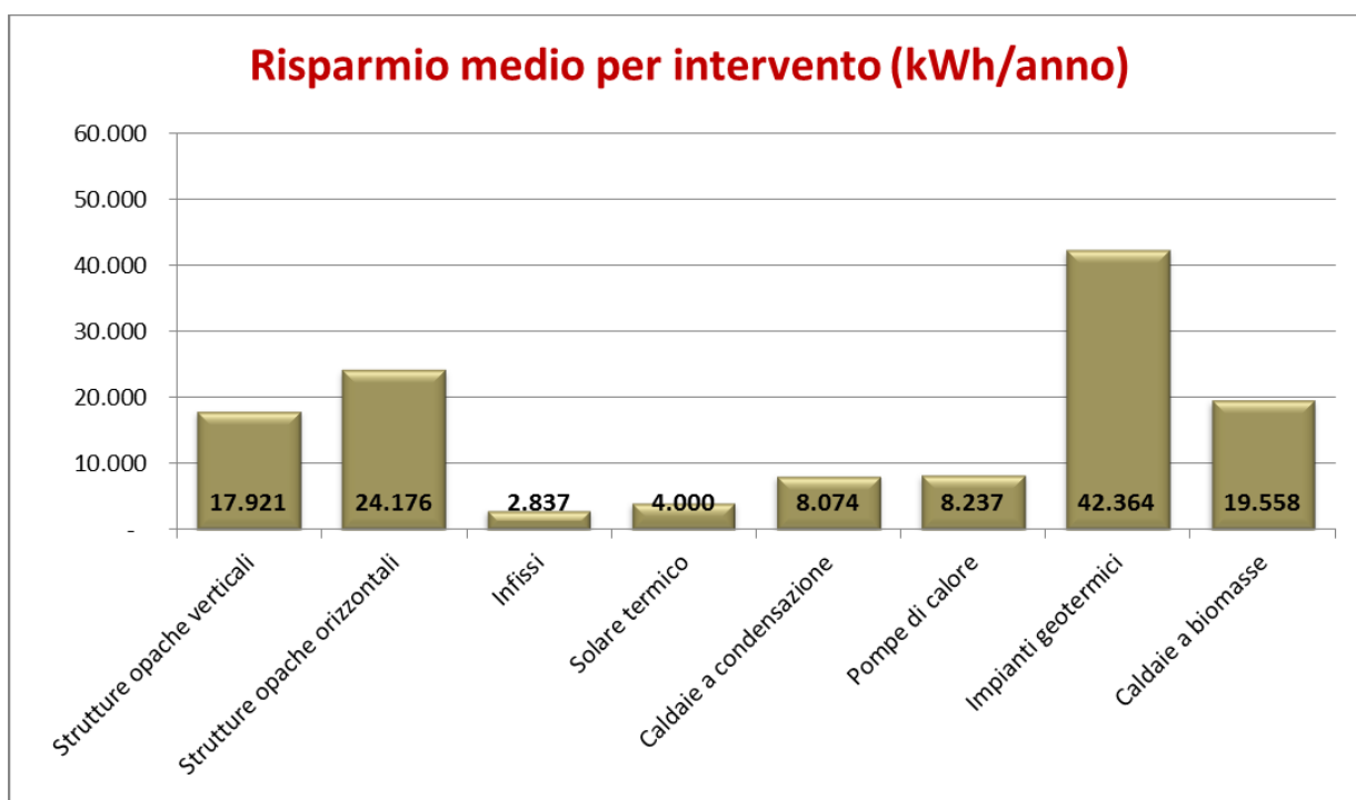
FIG. 10 RISPARMIO MEDIO ANNUO ASSOCIATO ALLA SINGOLA TIPOLOGIA DI INTERVENTO. VALORI ESPRESSI IN kWh/ANNO – REGIONE FRIULI-VENEZIA GIULIA, ANNO 2014
