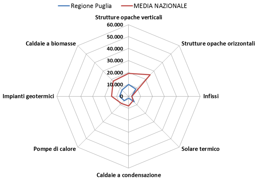
FIG. 15 RISPARMIO MEDIO ANNUO PER TIPOLOGIA DI INTERVENTO IN RAPPORTO ALLA MEDIA NAZIONALE. VALORI ESPRESSI IN kWh/ANNO – REGIONE PUGLIA, ANNO 2014
