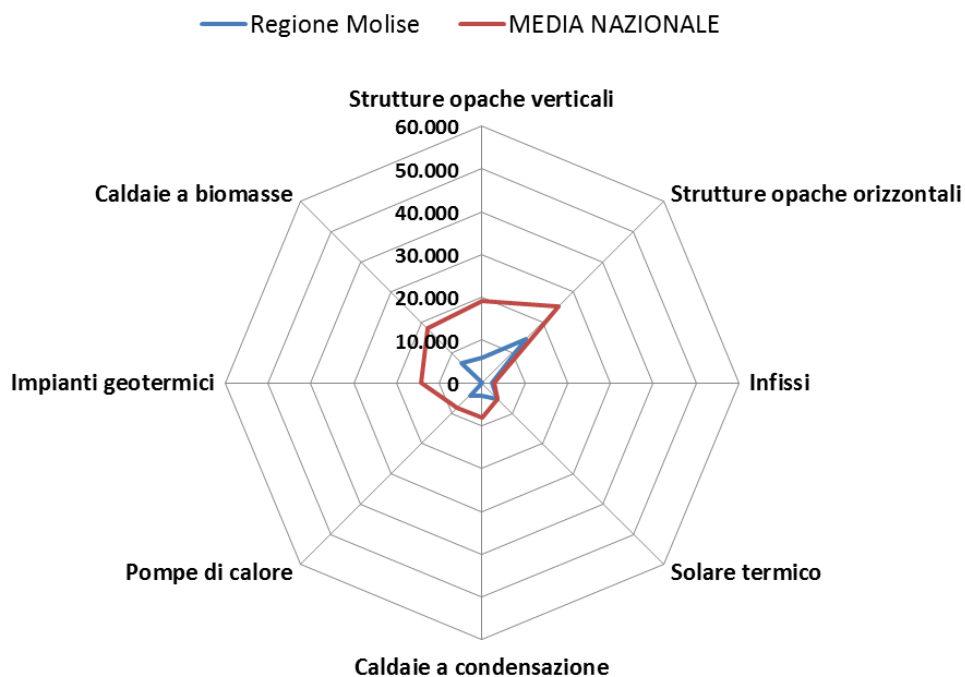
FIG. 15 RISPARMIO MEDIO ANNUO PER TIPOLOGIA DI INTERVENTO IN RAPPORTO ALLA MEDIA NAZIONALE. VALORI ESPRESSI IN kWh/ANNO – REGIONE MOLISE, ANNO 2014
