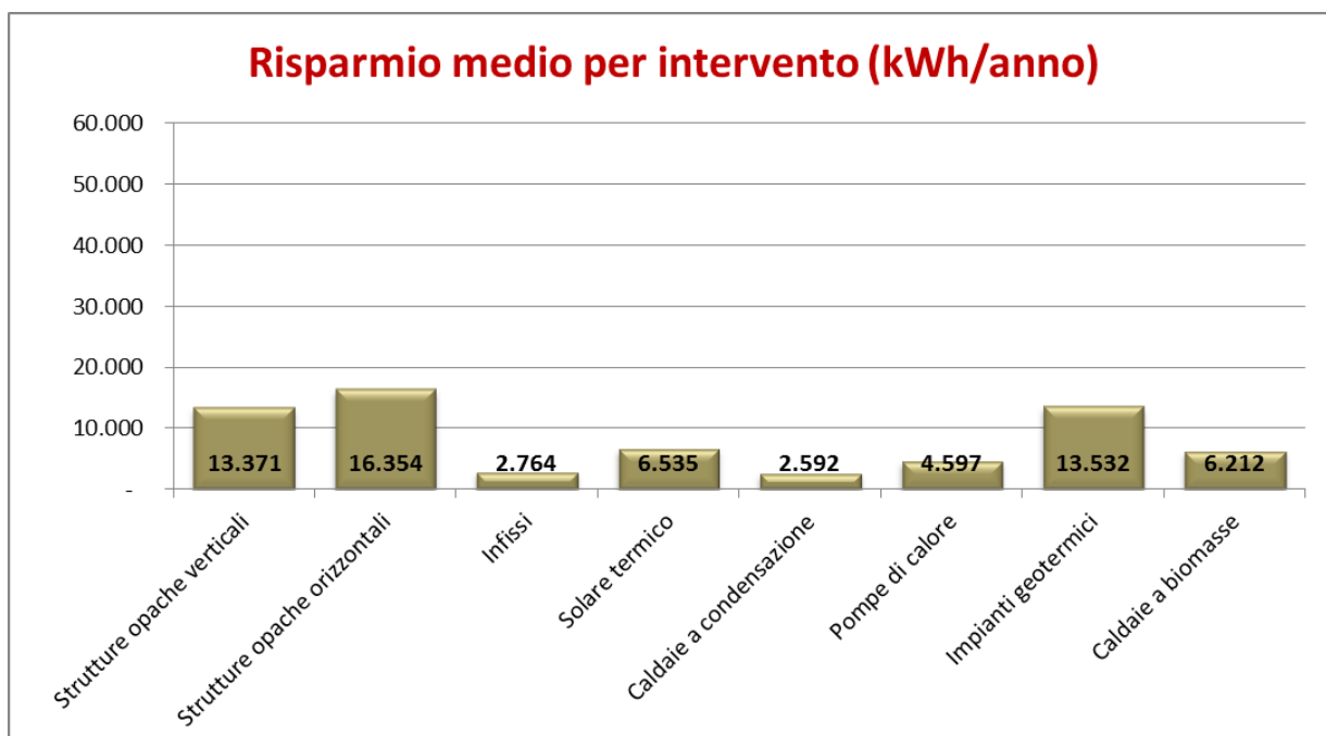
FIG. 10 RISPARMIO MEDIO ANNUO ASSOCIATO ALLA SINGOLA TIPOLOGIA DI INTERVENTO. VALORI ESPRESSI IN kWh/ANNO – REGIONE ABRUZZO, ANNO 2014
