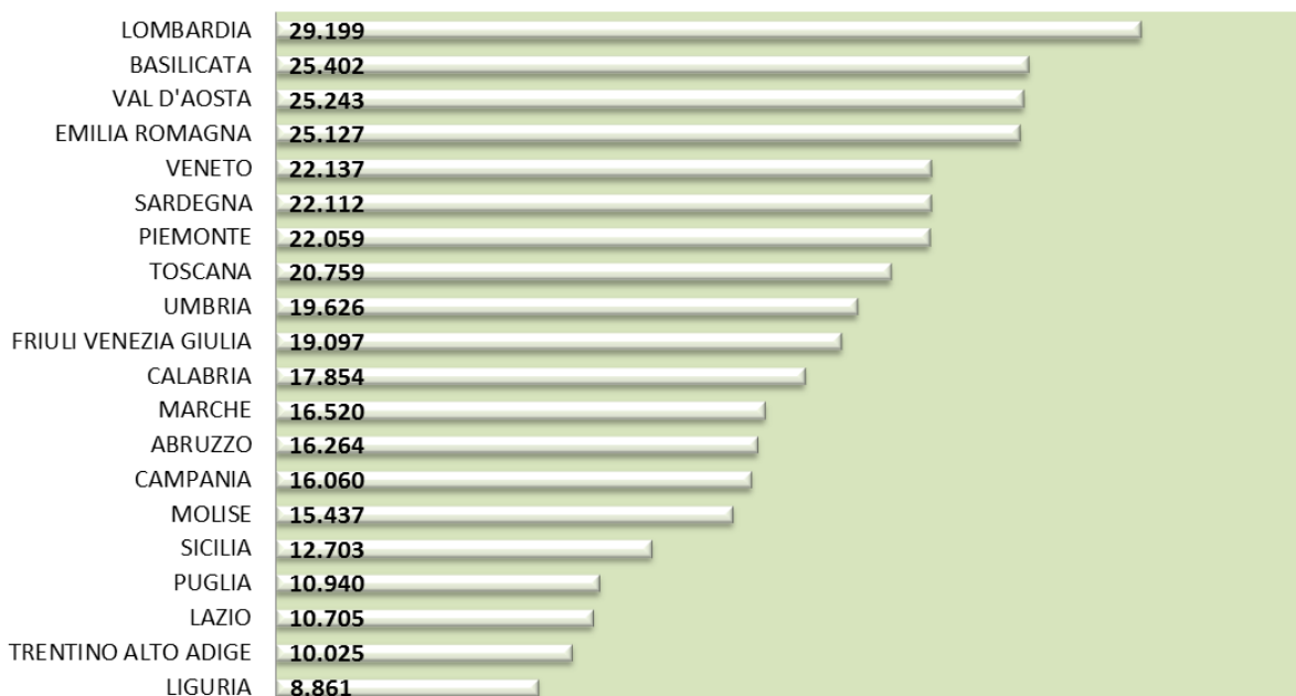
FIG.4.4 INTERVENTI SU STRUTTURE OPACHE ORIZZONTALI. RISPARMIO REALIZZATO CON L'INTERVENTO MEDIO EFFETTUATO NEL 2014. DATO NORMALIZZATO IN FUNZIONE DEI GRADI GIORNO REGIONALI (kWh/ANNO)
