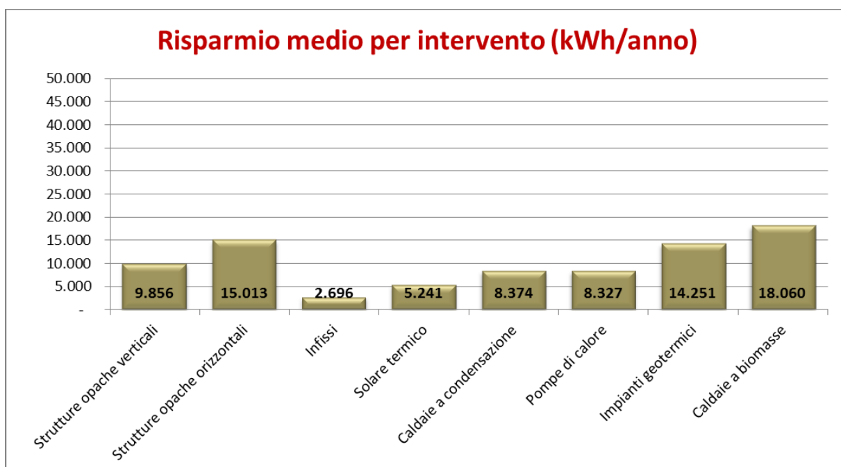
FIG. 14 RISPARMIO MEDIO ANNUO OTTENUTO PER TIPOLOGIA DI INTERVENTO. DATI ESPRESSI IN kWh/ANNO – ITALIA, ANNO 2014
