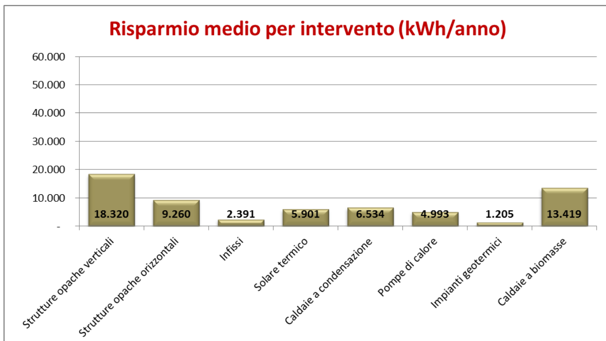
FIG. 10 RISPARMIO MEDIO ANNUO ASSOCIATO ALLA SINGOLA TIPOLOGIA DI INTERVENTO. VALORI ESPRESSI IN kWh/ANNO – REGIONE LAZIO, ANNO 2014
