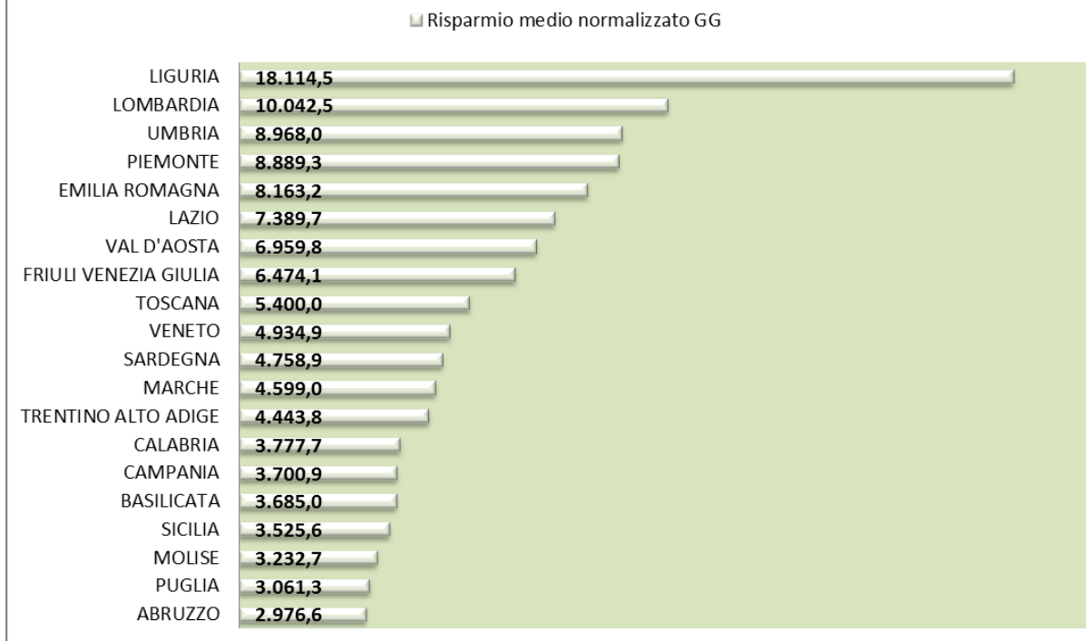
FIG.6.4 SOSTITUZIONE DI IMPIANTI TERMICI. RISPARMIO REALIZZATO CON L'INTERVENTO MEDIO EFFETTUATO NEL 2014. DATO NORMALIZZATO IN FUNZIONE DEI GRADI GIORNO REGIONALI (kWh/ANNO)
