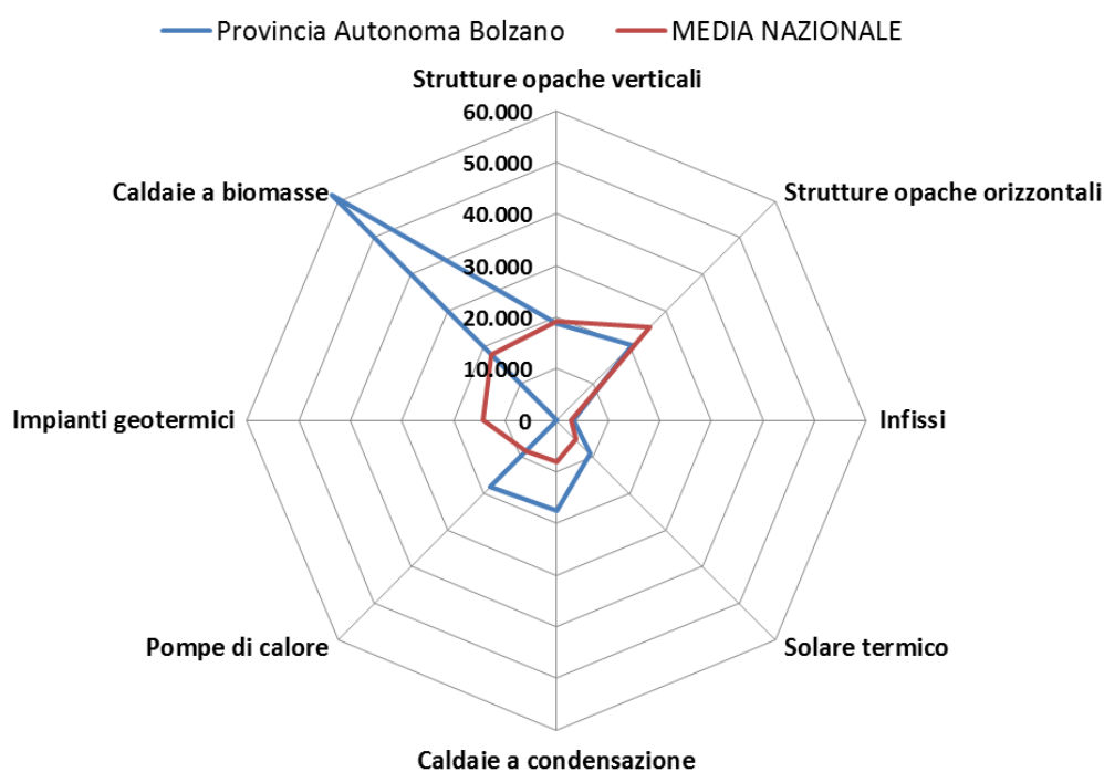
FIG. 15 RISPARMIO MEDIO ANNUO PER TIPOLOGIA DI INTERVENTO IN RAPPORTO ALLA MEDIA NAZIONALE. VALORI ESPRESSI IN kWh/ANNO – REGIONE TRENTINO-ALTO ADIGE PROVINCIA AUTONOMA DI BOLZANO, ANNO 2014
