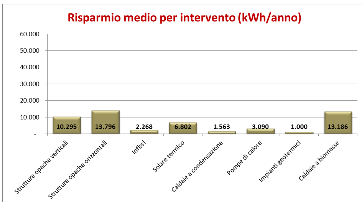
FIG. 10 RISPARMIO MEDIO ANNUO ASSOCIATO ALLA SINGOLA TIPOLOGIA DI INTERVENTO. VALORI ESPRESSI IN kWh/ANNO – REGIONE SARDEGNA, ANNO 2014
