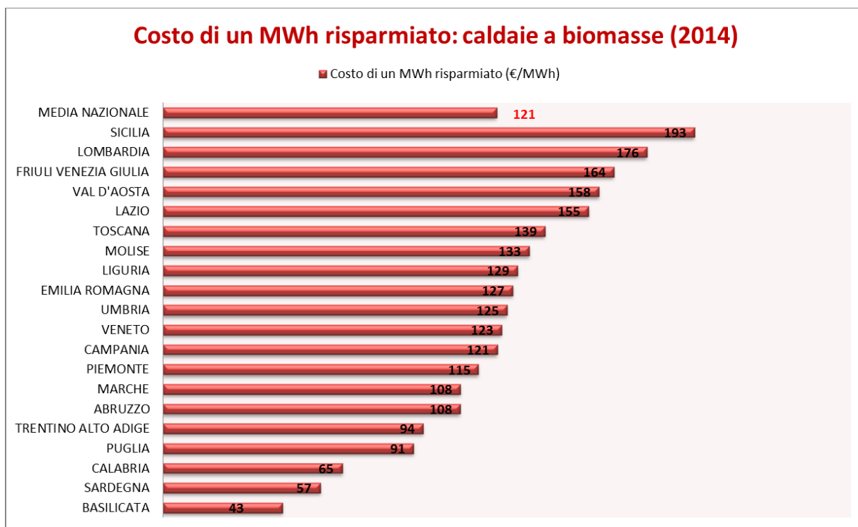
FIG.3.5 SOSTITUZIONE DI IMPIANTI TERMICI CON CALDAIE A BIOMASSE. COSTO MEDIO DI UN MWh RISPARMIATO A SEGUITO DEGLI INTERVENTI EFFETTUATI NEL 2014
