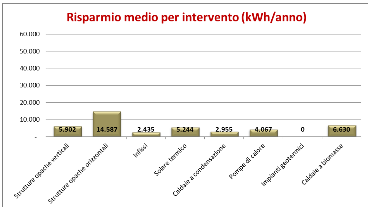
FIG. 10 RISPARMIO MEDIO ANNUO ASSOCIATO ALLA SINGOLA TIPOLOGIA DI INTERVENTO. VALORI ESPRESSI IN kWh/ANNO – REGIONE MOLISE, ANNO 2014
