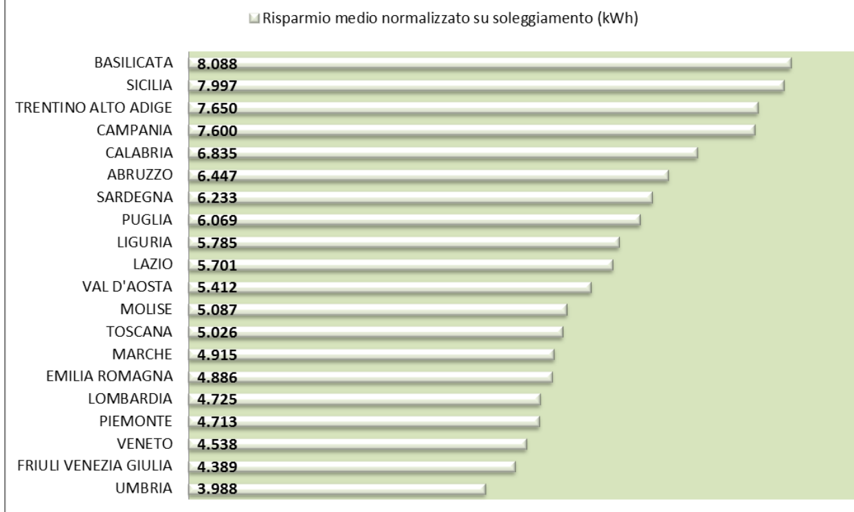
FIG.5.5 SOLARE TERMICO. RISPARMIO REALIZZATO CON L'INTERVENTO MEDIO EFFETTUATO NEL 2014. DATO NORMALIZZATO IN FUNZIONE DEL VALORE DI SOLEGGIAMENTO MEDIO (kWh/ANNO)
