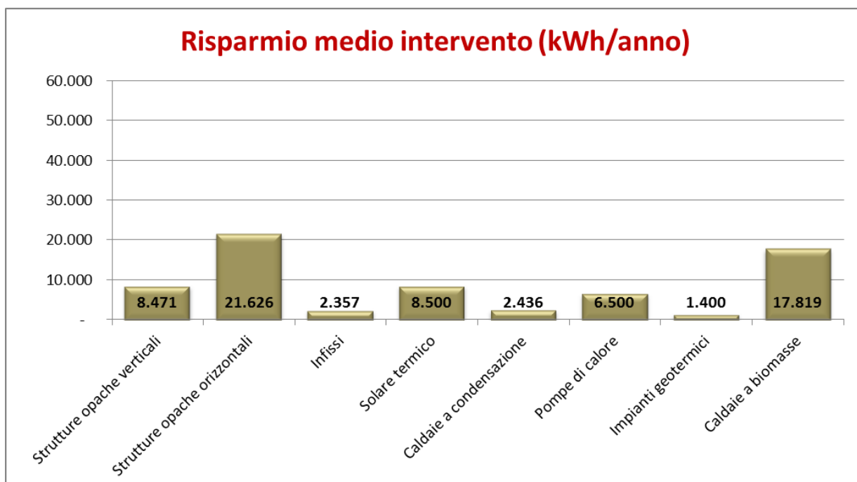
FIG. 10 RISPARMIO MEDIO ANNUO ASSOCIATO ALLA SINGOLA TIPOLOGIA DI INTERVENTO. VALORI ESPRESSI IN kWh/ANNO – REGIONE BASILICATA, ANNO 2014
