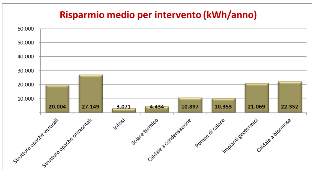
FIG. 10 RISPARMIO MEDIO ANNUO ASSOCIATO ALLA SINGOLA TIPOLOGIA DI INTERVENTO. VALORI ESPRESSI IN kWh/ANNO – REGIONE PIEMONTE, ANNO 2014
