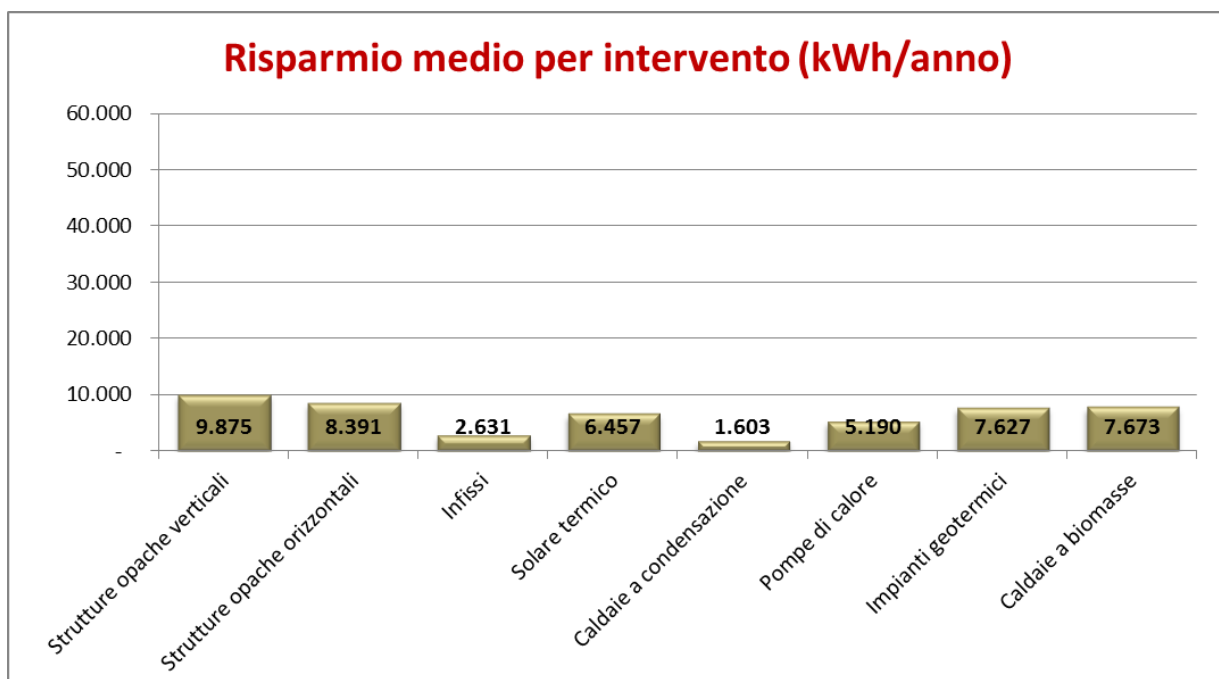
FIG. 10 RISPARMIO MEDIO ANNUO ASSOCIATO ALLA SINGOLA TIPOLOGIA DI INTERVENTO. VALORI ESPRESSI IN kWh/ANNO – REGIONE PUGLIA, ANNO 2014
