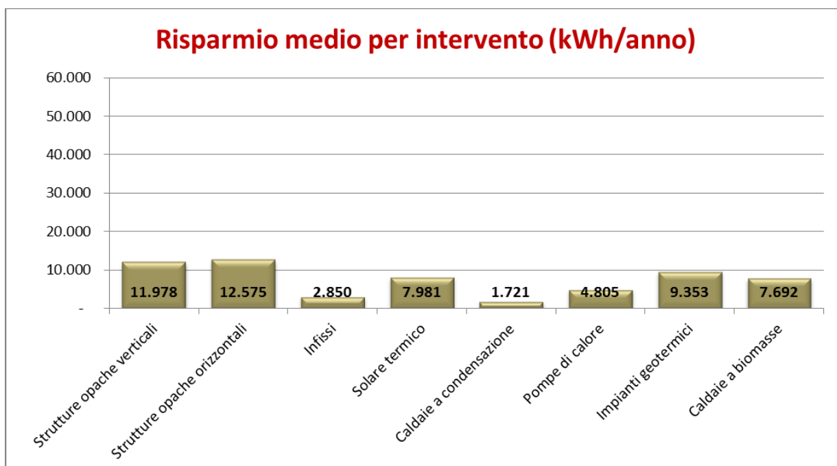
FIG. 10 RISPARMIO MEDIO ANNUO ASSOCIATO ALLA SINGOLA TIPOLOGIA DI INTERVENTO. VALORI ESPRESSI IN kWh/ANNO – REGIONE CAMPANIA, ANNO 2014
