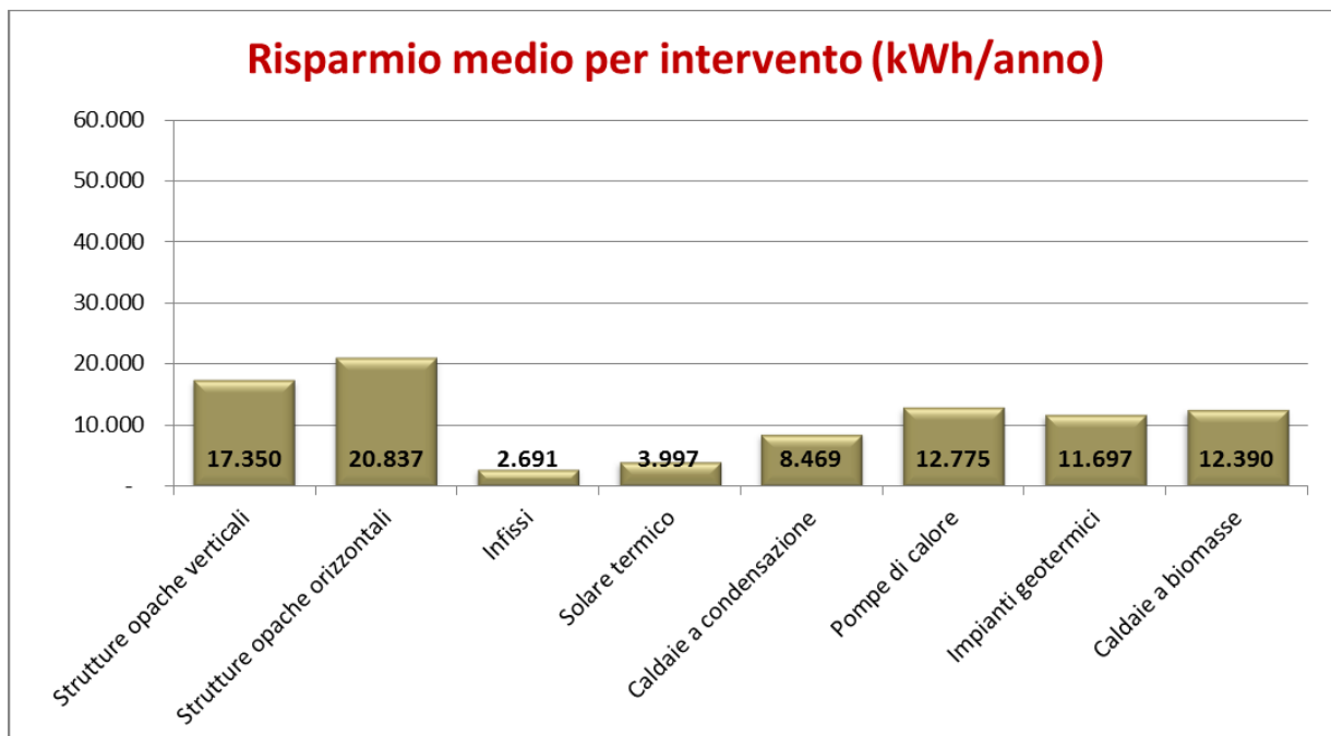
FIG. 10 RISPARMIO MEDIO ANNUO ASSOCIATO ALLA SINGOLA TIPOLOGIA DI INTERVENTO. VALORI ESPRESSI IN kWh/ANNO – REGIONE UMBRIA, ANNO 2014
