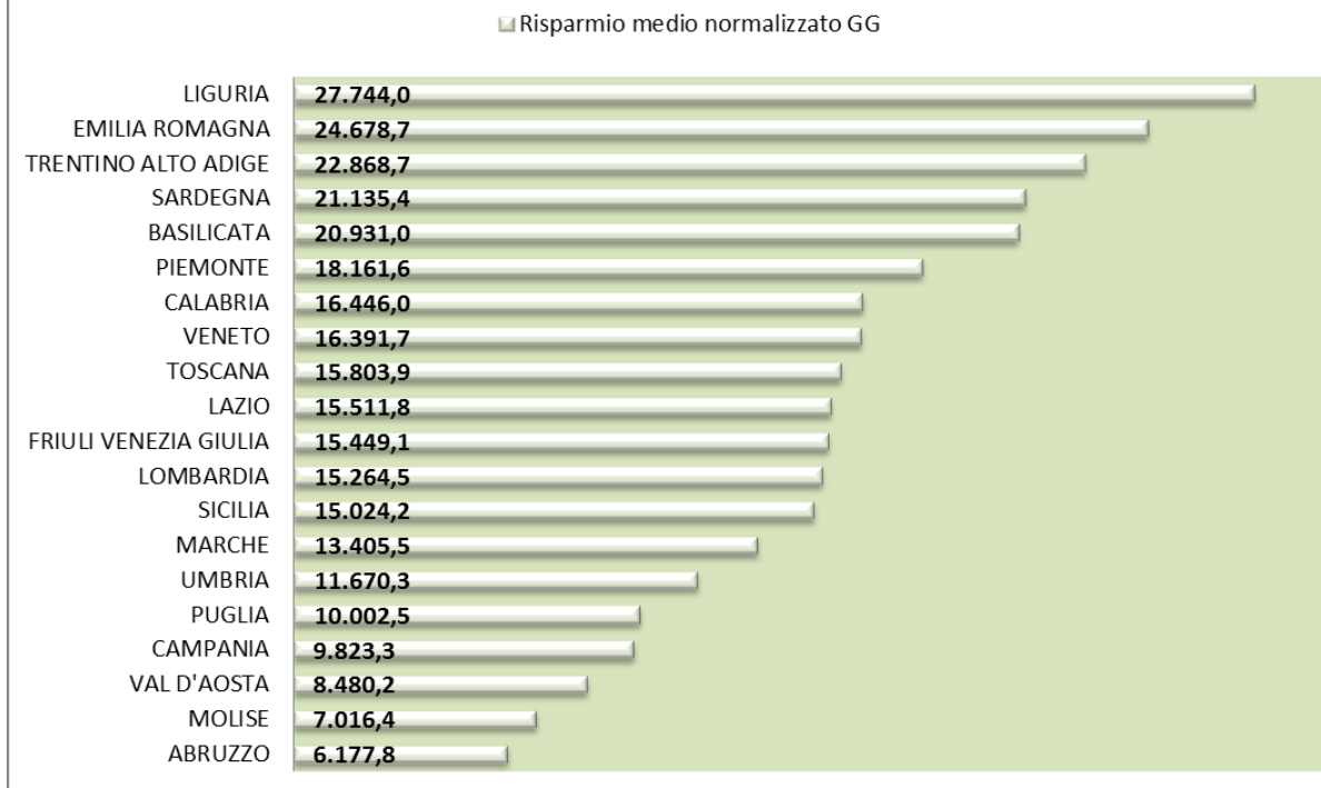
FIG. 3.3 SOSTITUZIONE DI IMPIANTI TERMICI CON CALDAIE A BIOMASSE. RISPARMIO REALIZZATO CON L'INTERVENTO MEDIO EFFETTUATO NEL 2014. DATO NORMALIZZATO IN FUNZIONE DEI GRADI GIORNO REGIONALI (kWh/ANNO)
