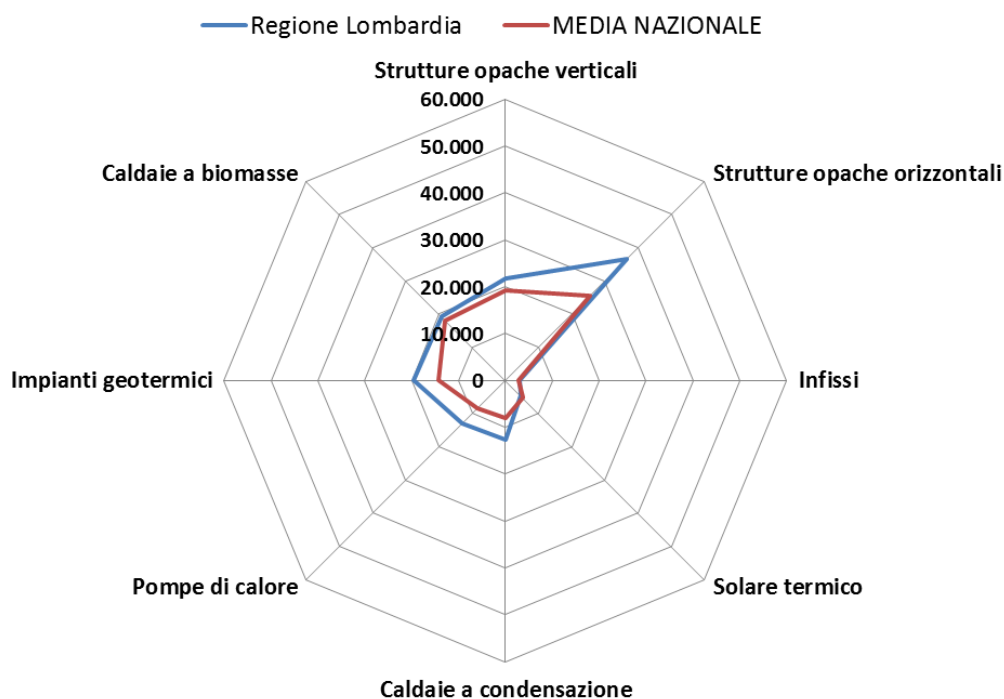
FIG. 15 RISPARMIO MEDIO ANNUO PER TIPOLOGIA DI INTERVENTO IN RAPPORTO ALLA MEDIA NAZIONALE. VALORI ESPRESSI IN kWh/ANNO – REGIONE LOMBARDIA, ANNO 2014
