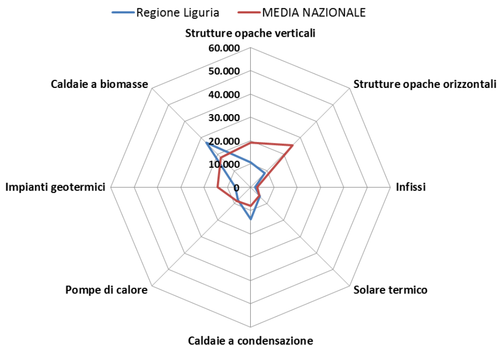
FIG. 15 RISPARMIO MEDIO ANNUO PER TIPOLOGIA DI INTERVENTO IN RAPPORTO ALLA MEDIA NAZIONALE. VALORI ESPRESSI IN kWh/ANNO – REGIONE LIGURIA, ANNO 2014
