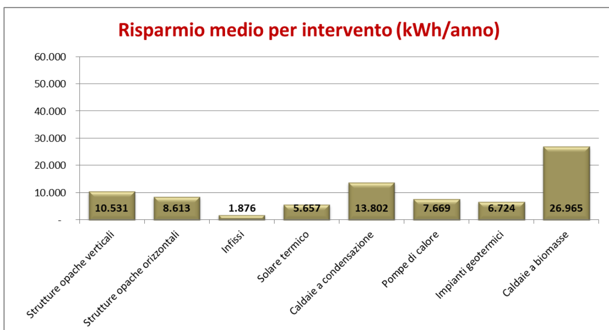
FIG. 10 RISPARMIO MEDIO ANNUO ASSOCIATO ALLA SINGOLA TIPOLOGIA DI INTERVENTO. VALORI ESPRESSI IN kWh/ANNO – REGIONE LIGURIA, ANNO 2014
