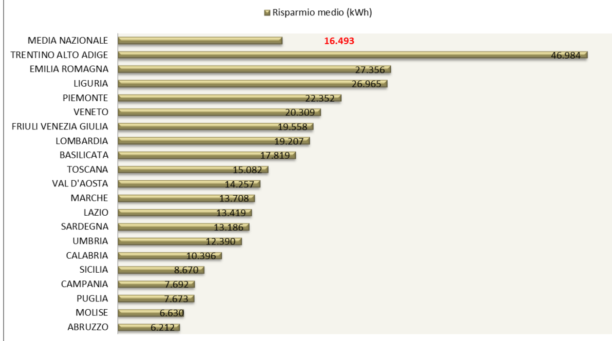
FIGURA 3.2 SOSTITUZIONE DI IMPIANTI TERMICI CON CALDAIE A BIOMASSE. RISPARMIO REALIZZATO CON L'INTERVENTO MEDIO EFFETTUATO NEL 2014 (kWh/ANNO)
