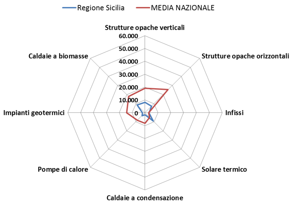
FIG. 15 RISPARMIO MEDIO ANNUO PER TIPOLOGIA DI INTERVENTO IN RAPPORTO ALLA MEDIA NAZIONALE. VALORI ESPRESSI IN kWh/ANNO – REGIONE SICILIA, ANNO 2014
