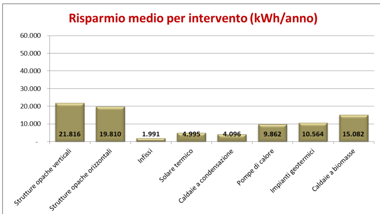
FIG. 10 RISPARMIO MEDIO ANNUO ASSOCIATO ALLA SINGOLA TIPOLOGIA DI INTERVENTO. VALORI ESPRESSI IN kWh/ANNO – REGIONE TOSCANA, ANNO 2014
