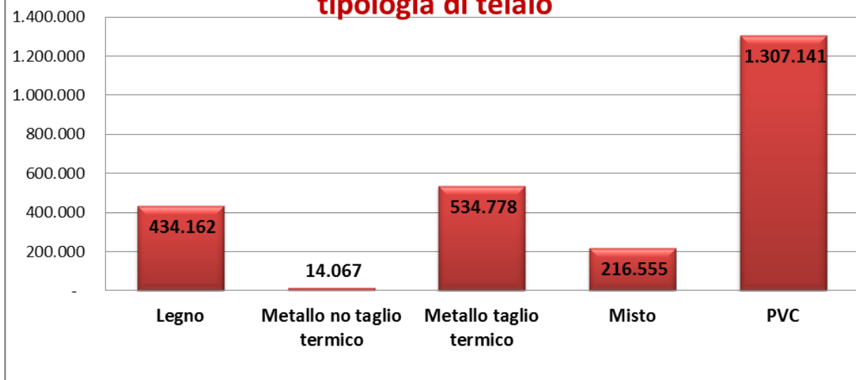
FIG. 4.25 METRI QUADRI TOTALI INSTALLATI NEL 2014 PER TIPOLOGIA DI TELAIO
