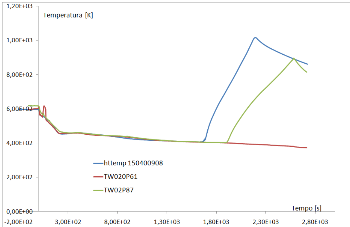
Fig.9: Andamento della temperatura di parete nella parte alta del canale scaldante.
