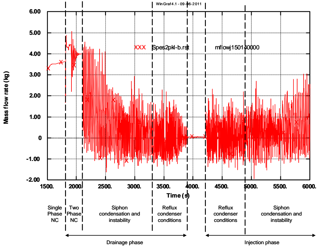
Fig.22: Portata attraverso il canale di potenza per l'esperimento su SPES2. Identificazione dei regimi instaurati.
