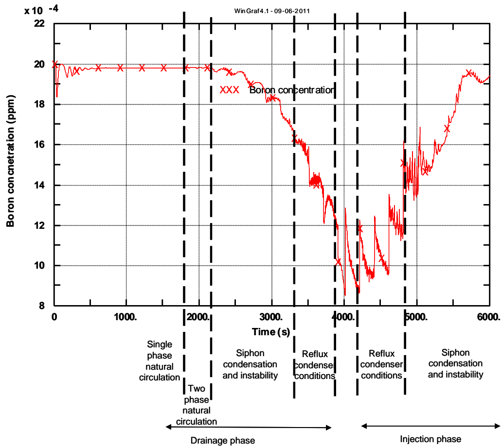
Fig. 23: Concentrazione di boro nel downcomer per l'esperimento su SPES2.
