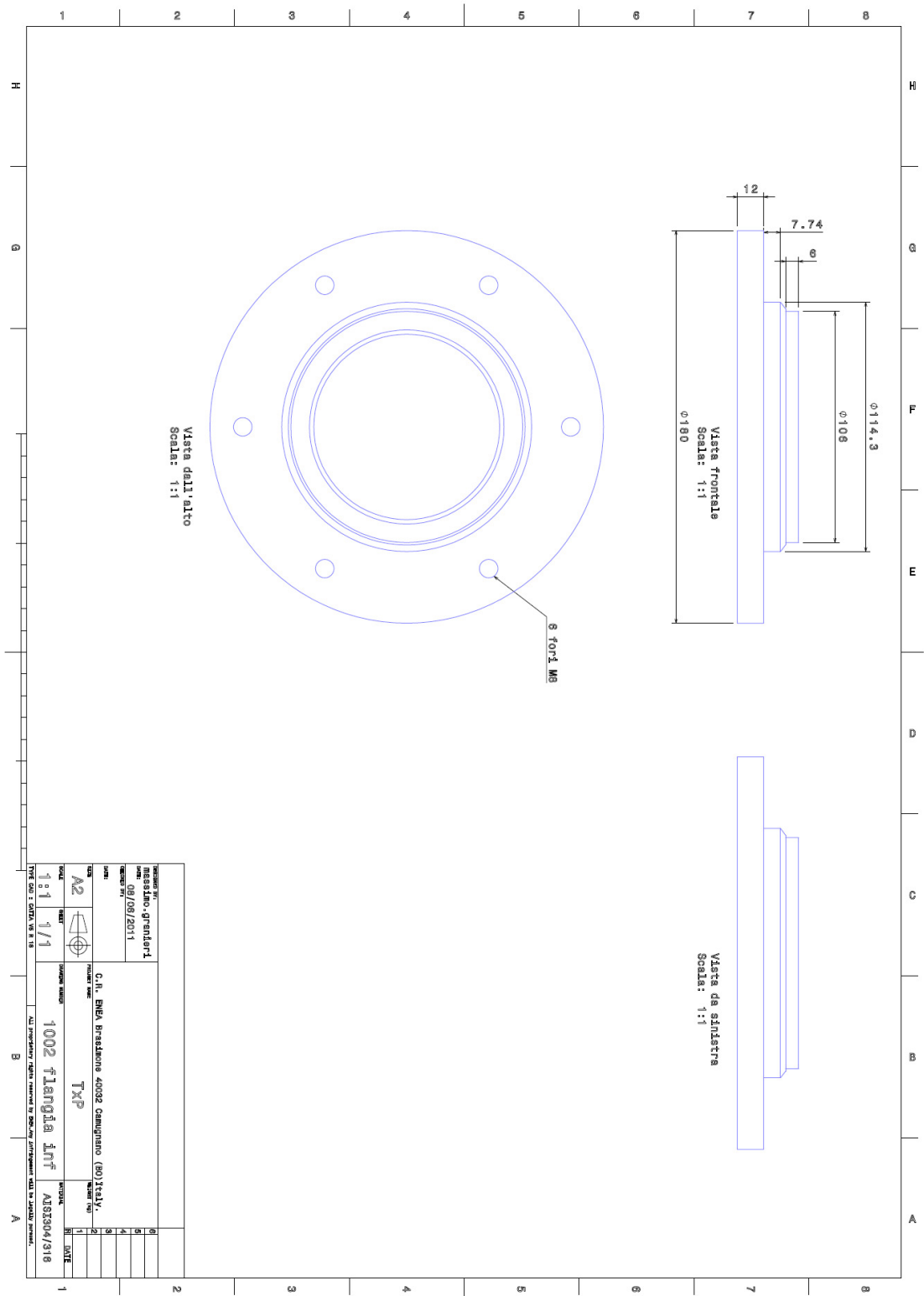
Fig. 41 – TxP design: PT bottom flange.
