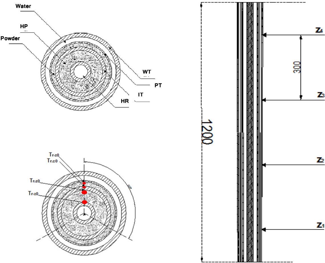
Fig. 5 – TxP instrumentation scheme.
