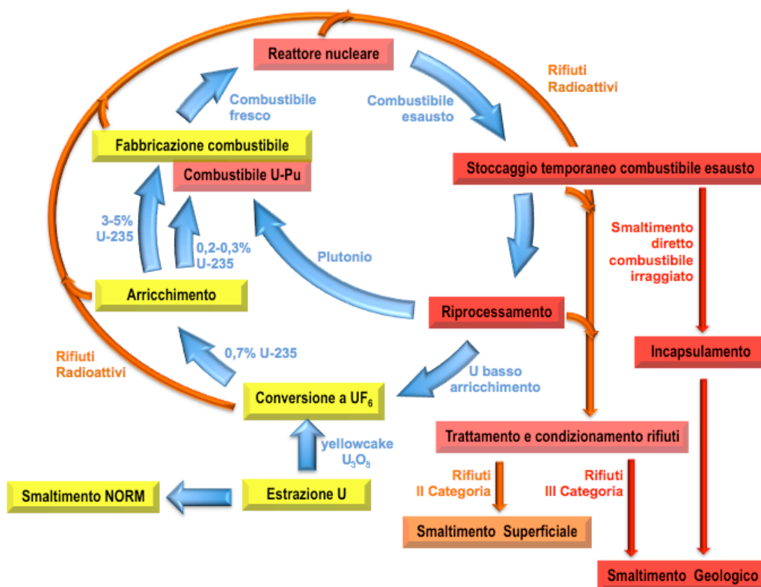
Figura 4.3.1: Rappresentazione schematica del ciclo del combustibile nucleare
