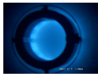
Impianto di irraggiamento γ CALLIOPE, che può essere utilizzato per irraggiamenti gamma di rilevanza scientifica e industriale. Rastrelliera dell'impianto con sorgenti di 60 Co e visione dell'effetto Cherenkov
