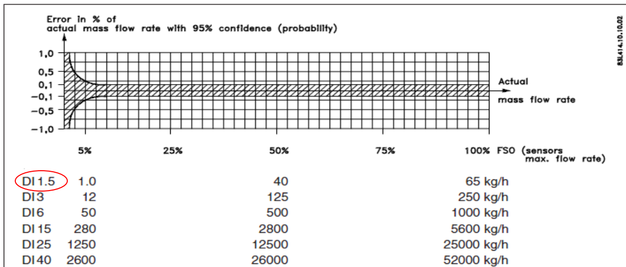
Figura 5-curva dell'errore
