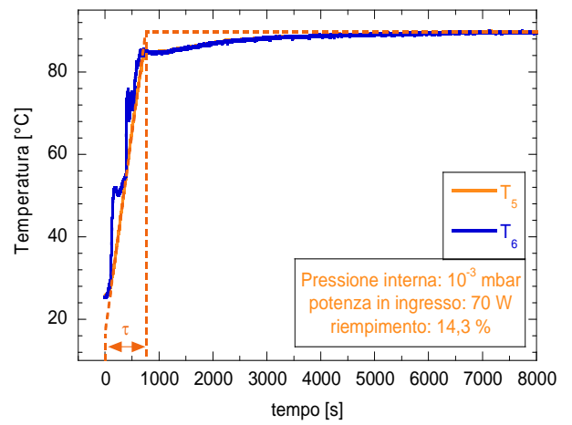
Figura 5-andamento di T per FR=14,3 %
