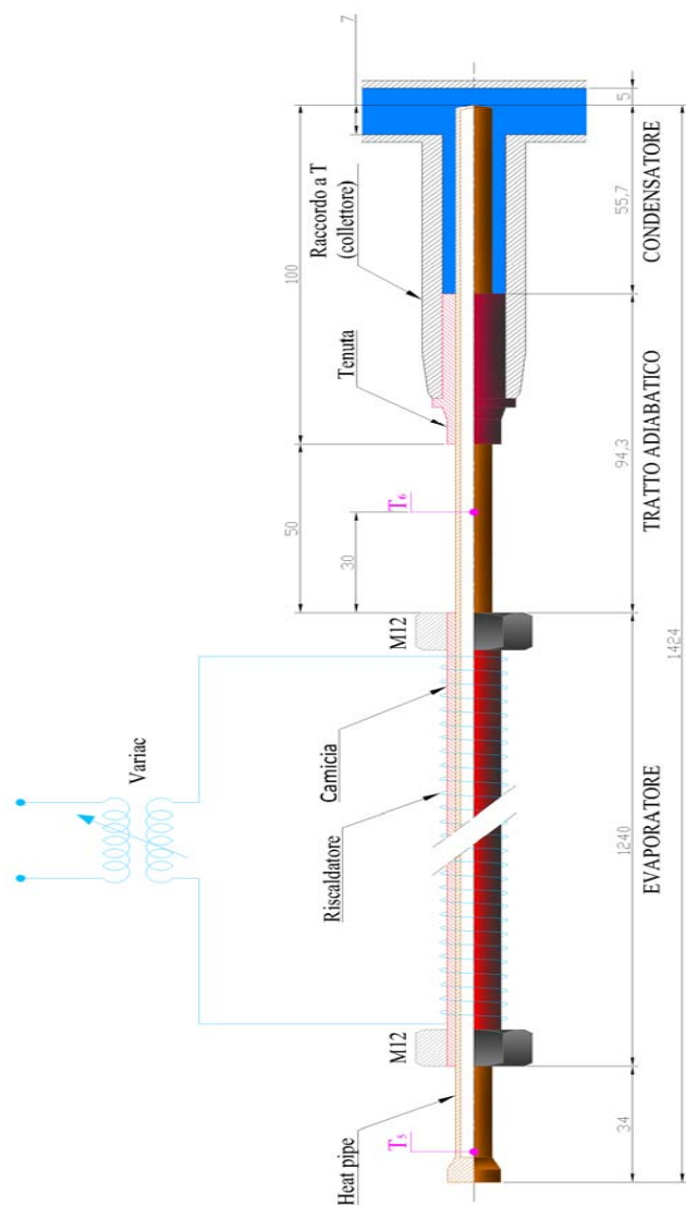
Figura 14-schema realizzativo dell'heat-pipe e dalla camicia esterna
