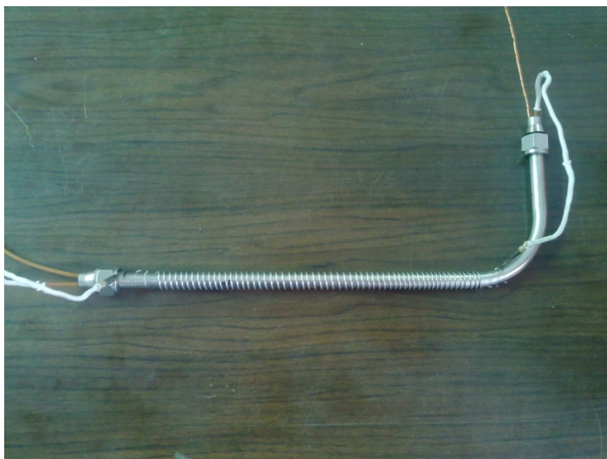
Figura 31-preriscaldatore senza coibentazione
