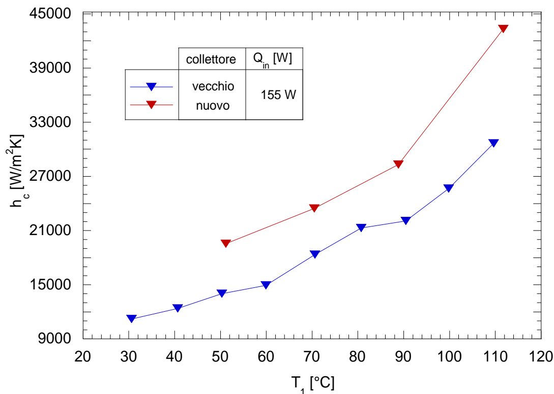
Figura 18 – andamento di h_c in funzione di T_1
