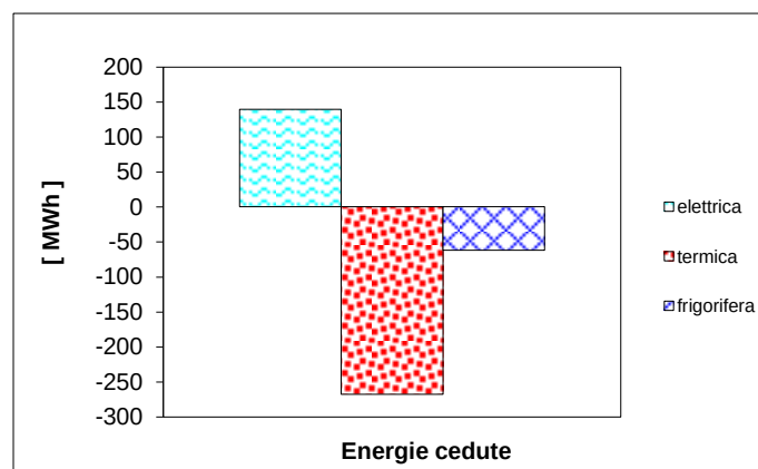
Fig. 66 – Variazione delle produzioni annue per intervento d’efficienza energetica
