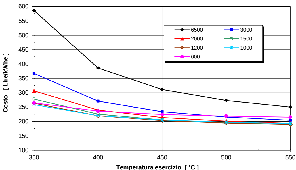
Fig. 190 – Costo medio dell'energia elettrica prodotta in funzione della temperatura di esercizio per diverse capacità d'accumulo
