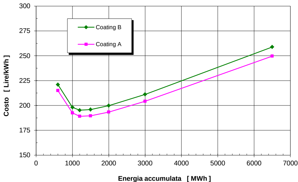
Fig. 192 – Costo medio dell'energia elettrica prodotta con i due tipi di rivestimento in funzione della capacità dell'accumulo
