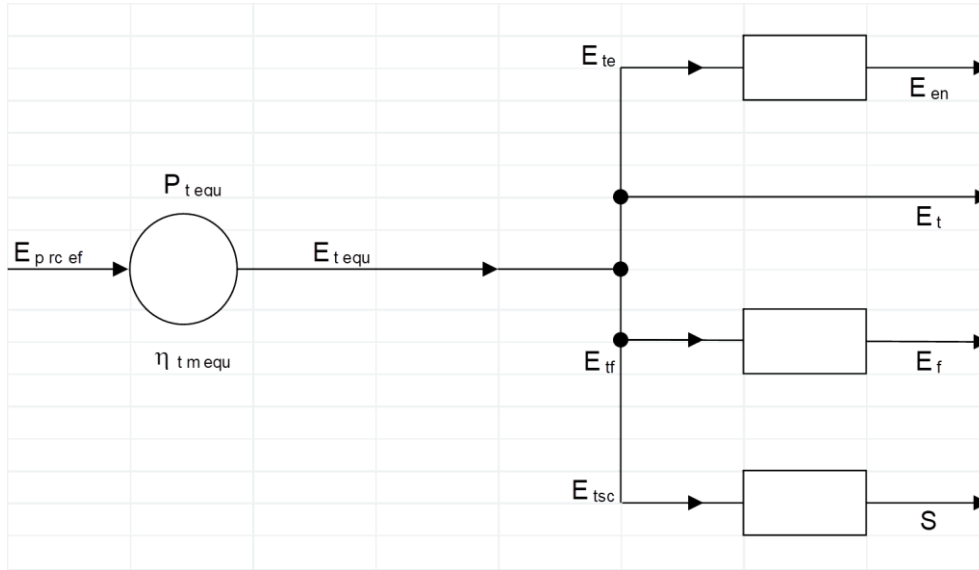
Fig. 167 – Schema equivalente dell'impianto di produzione combinata
