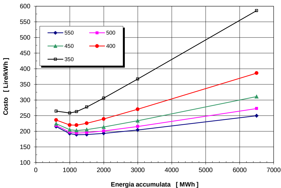
Fig. 191 – Costo medio dell'energia elettrica prodotta in funzione della capacità dell'accumulo termico per diverse temperature d'esercizio
