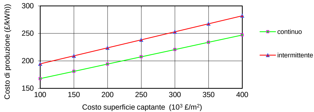
Fig. 181 – Influenza del costo unitario del campo solare sul costo di produzione
