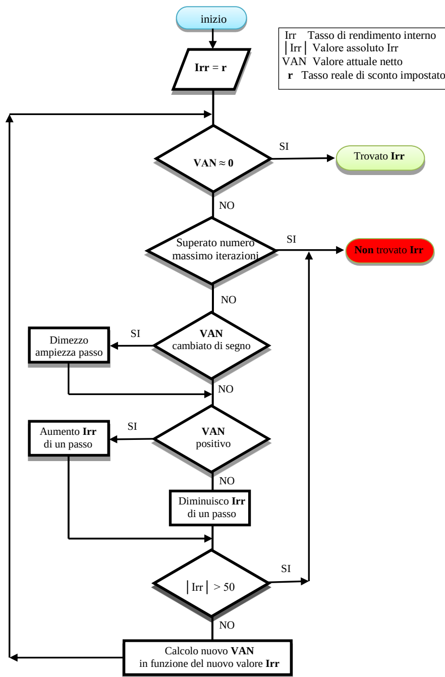
Fig. 242 – Diagramma di flusso dell'algoritmo per il calcolo dell'IRR
