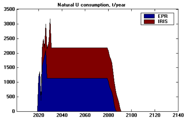
Grafico n. 6. Consumo cumulato di Uranio, t/anno (Scenario 4)
