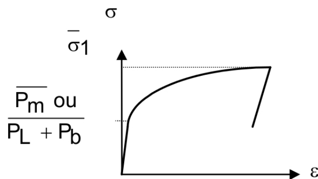
Figura 5.8: Metodo 1a per l'analisi elasto-plastica
