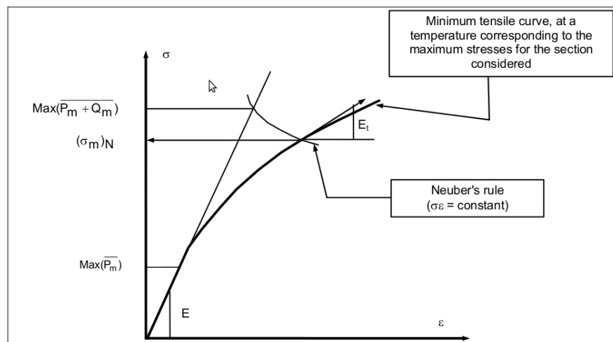
Figura 5.4: Determinazione grafica di (\sigma_m)_N e di E_t
