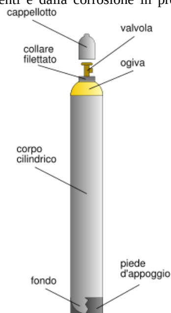
Figura 17.2 – Parti costituenti una bombola di gas compresso
