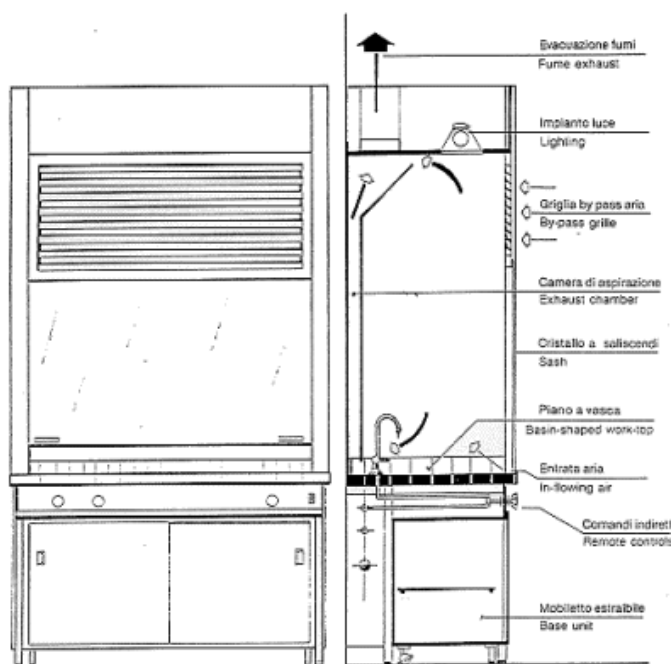
Figura 20.4 – Cappa con by pass d'aria
