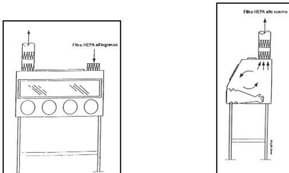
Figura 21.3 – Cappa biologica di classe III
