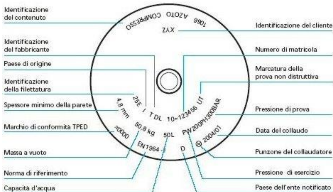
Figura 17.7 - Punzonatura dell'ogiva, significato
