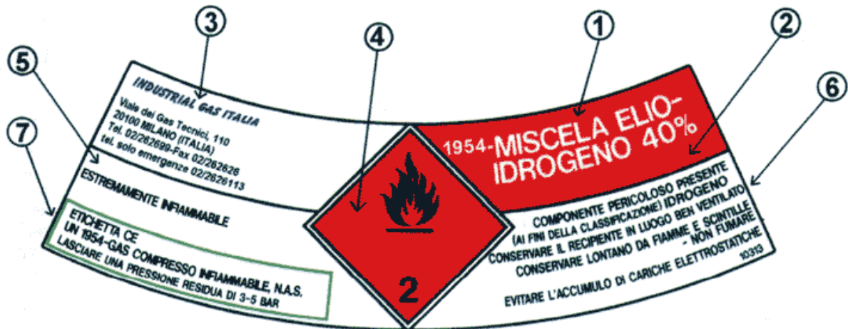
Figura 17.6 - Esempi di etichettatura dell'ogiva delle bombole
