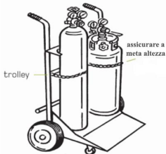
Figura 17.8 - Carrello portabombole
