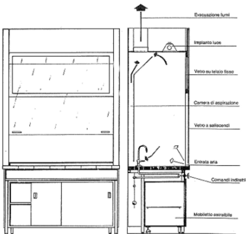
Figura 20.2 – Componenti di una cappa chimica ad espulsione d'aria
