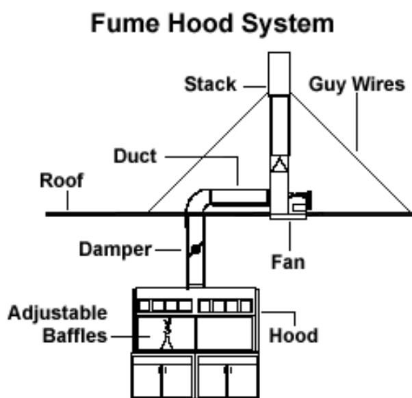
Figura 20.1 – Cappe chimiche ad espulsione di aria
