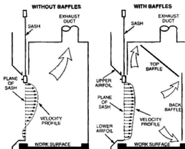
Figura 20.3 – Differenza fra cappa ad un solo punto di aspirazione e cappa a più punti di aspirazione
