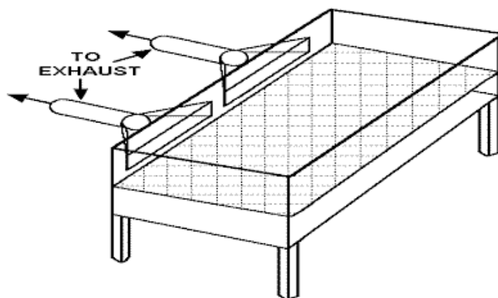
Figura 20.11 – Piano di lavoro aspirato
