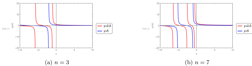
Fig. 3. Eqs. (4.9)–(4.10) vs. x for fixed y values.
