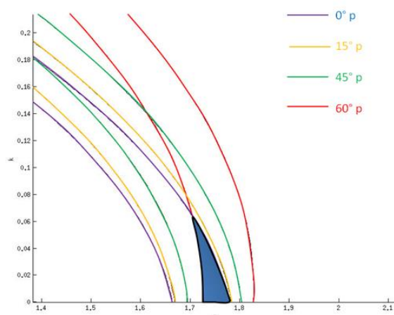
Figura 140. Range di n e k compatibili con i valori di trasmittanza sperimentali
