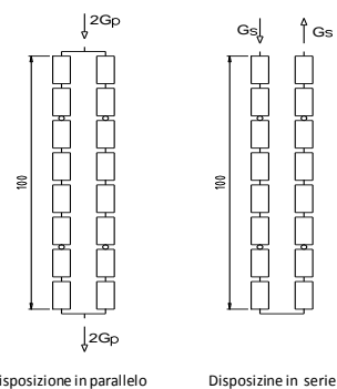
Figura 187. Possibili configurazioni dei collettori nel campo solare
