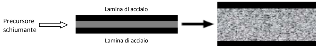
Figura 550. Realizzazione di AFS con pelli in AISI 316L e precursore AlSi_{10}
