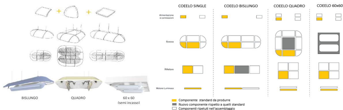
Figura 398. Schema tecnico COEELO
