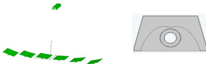
Figura 447. Immagine 3D del concentratore a specchi lineari di Fresnel e dettaglio del ricevitore in sezione
