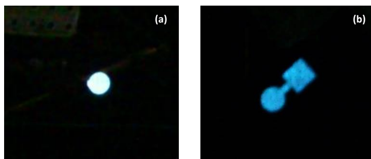
Figura 378. Fotografie di OLED utilizzanti (a) blend PVK:TAT 1b 5:1, (b) PFO:TAT 1b di 5:2
