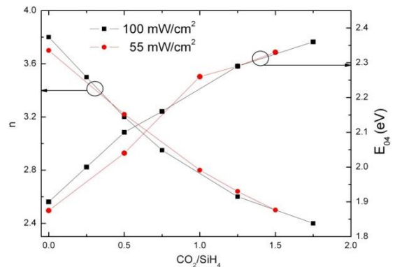
Figura 127. Indice di rifrazione a 635 nm e E_{04} valutati per le serie cresciute a 55 e 100 mW/cm 2
