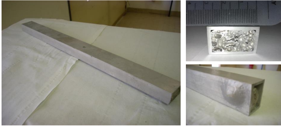
Figura 549. Profilato estruso di lunghezza 400 mm con evidenza della zona di collasso per eccessiva vicinanza alla parete posteriore del forno
