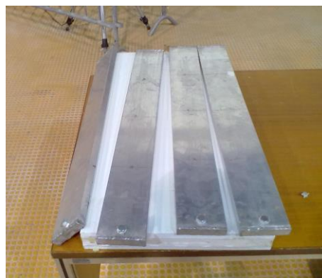
Figura 385. Pannello con PCM dopo il test su tavola
