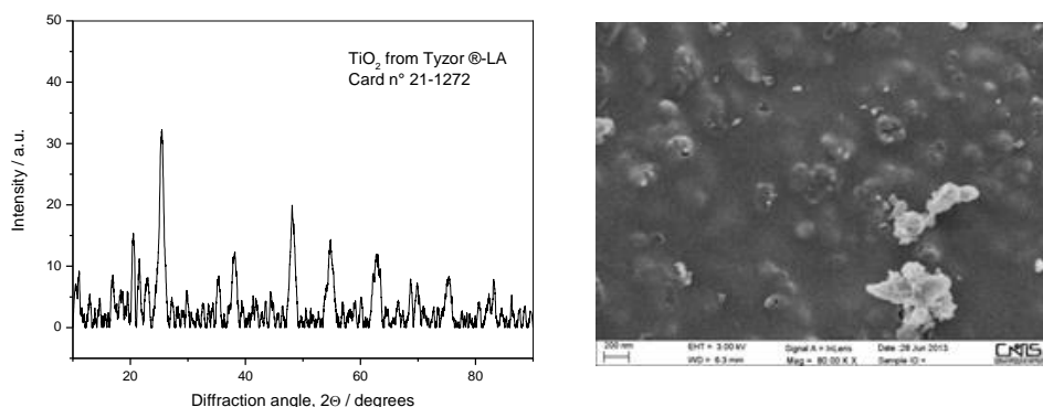
Figura 27. Diffratogramma ai raggi X del campione di TOL-C e immagine SEM del materiale
