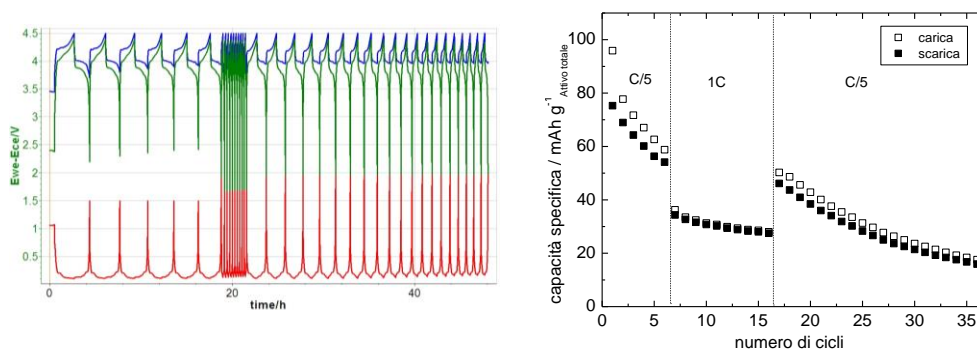
Figura 4. Profili di potenziale del catodo (blu), dell'anodo (rosso) e della batteria K14/SI-a20 (verde) in EC:DMC LiPF 6 1 M e i valori di capacità specifica della batteria riferiti al peso del materiale attivo totale durante i cicli di carica-scarica a C/5 e 1C
