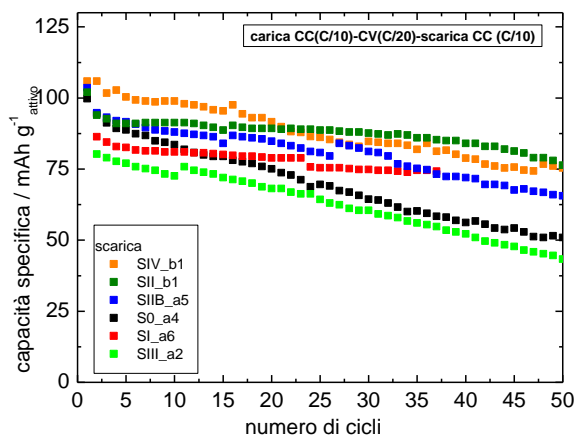
Figura 1. Confronto a 50°C della capacità specifica di scarica e vs. numero di cicli CC(C/10)-CV(C/20)/CC(C/10) fra 2,5 e 4,5 V di elettrodi di diversa tipologia
