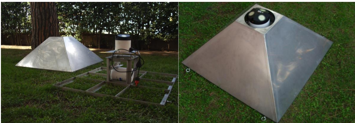
Figura 233. Struttura con profilatore acustico montato
