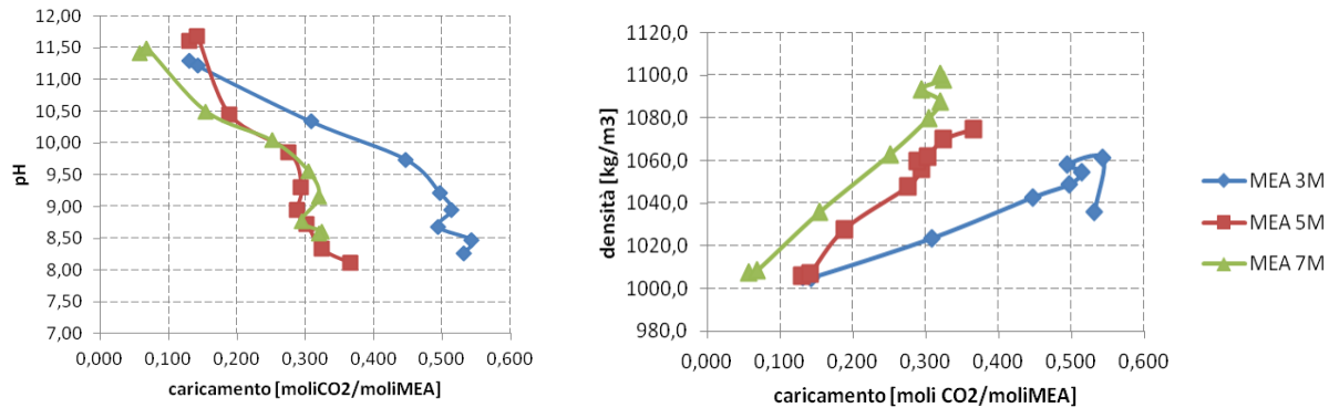
Figura 253. Andamento del pH e della densità in funzione del caricamento (moli CO 2 /moli MEA )
