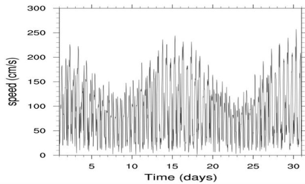
Figura 236. Velocità nel piano orizzontale della corrente di marea simulata dal modello numerico MITgcm durante un ciclo completo di marea. L'andamento temporale si riferisce al punto di griglia più vicino al punto considerato per la campagna di misure e a una profondità di 7 m
