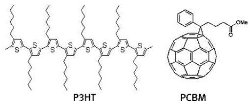
Figura 169. Struttura delle molecole di PH3T e di PCBM
