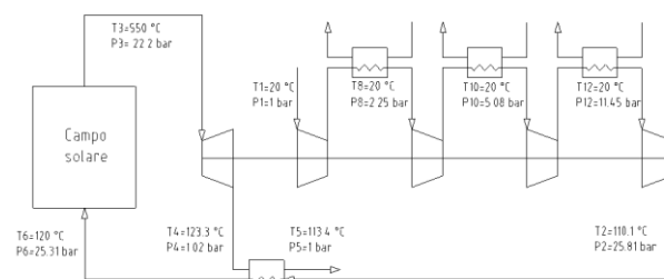
a) Ciclo aperto con rigenerazione e inter-refrigerazione
