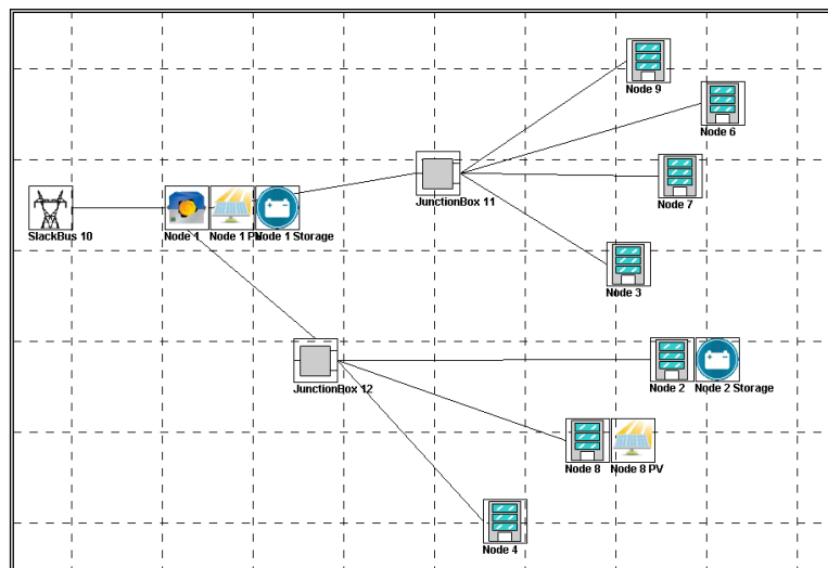
Figura 389. Esempio di topologia di rete elettrica con nodo di saldo, 2 nodi di generazione, 7 nodi di carico e 2 di giunzione. Nella topologia sono presenti anche dei componenti ausiliari quali pannelli fotovoltaici e sistemi di accumulo elettrico
