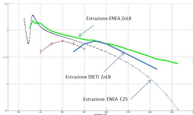
Figura 141. Comparazione tra spettri sperimentali ellissometrici dell'indice di rifrazione dello ZnO e valori ottenuti tramite estrazione effettuata dall'Università
