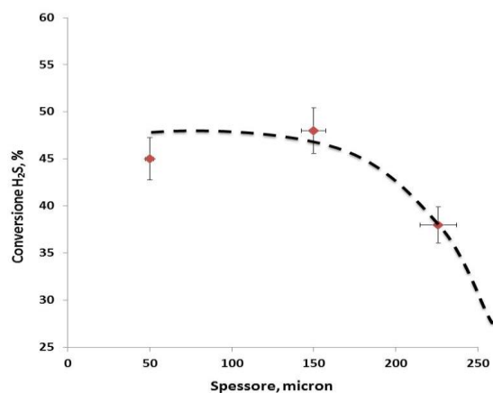
Figura 106. Determinazione dello spessore ottimale di washcoat ( O_2/H_2S = 0,5 ; T = 200 °C; Q = 800 Ncm^3/min )
