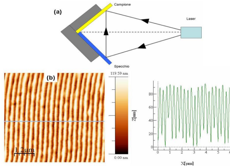
Figura 129. a) Configurazione alla Lloyd del setup di litografia interferenziale; b) reticolo unidimensionale ottenuto dall'esposizione di un film di fotoresist al pattern interferenziale
