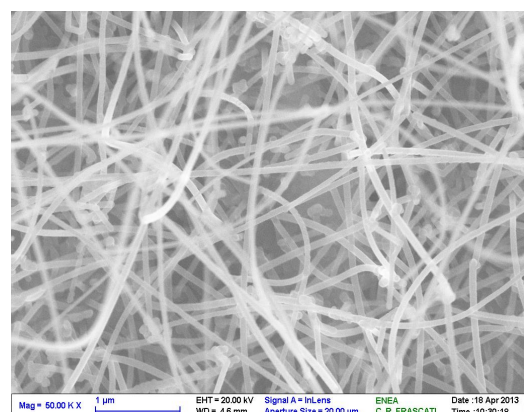
Figura 10. Foto SEM ad alto ingrandimento di SiNW/acciaio ottenuti mediante CVD a 618^\circ\text{C}
