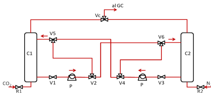
Figura 245. Schema dell'apparato sperimentale
