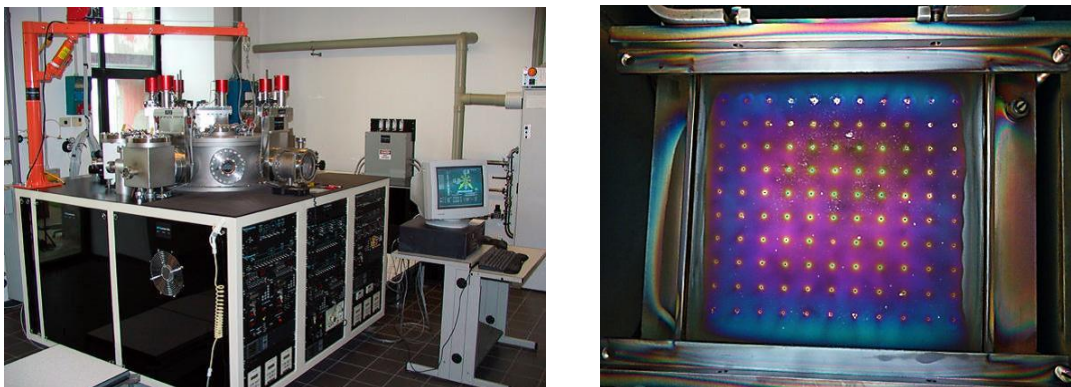
Figura 124. Impianto multicamera utilizzato per la fabbricazione di materiali e celle solari a film sottile ed elettrodo forellato utilizzato nella camera di deposizione dei film di silicio di tipo p
