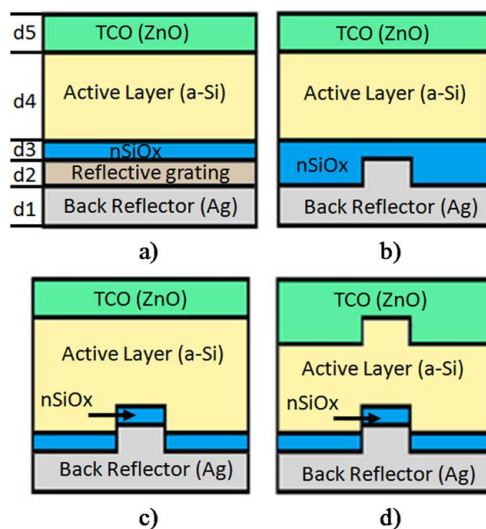
Figura 130. Schematizzazione delle configurazioni di celle solari analizzate
