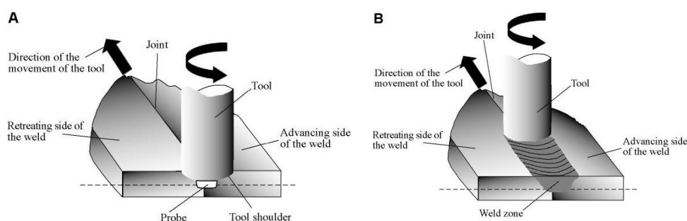
Figura 559 . Schematizzazione del processo di saldatura per FSW
