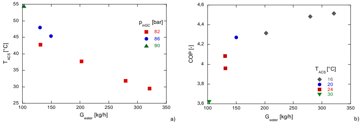
Figura 494. Temperatura dell'acqua in uscita dalla PdC al variare della portata erogata (a); COP della PdC in funzione della portata erogata (b)
