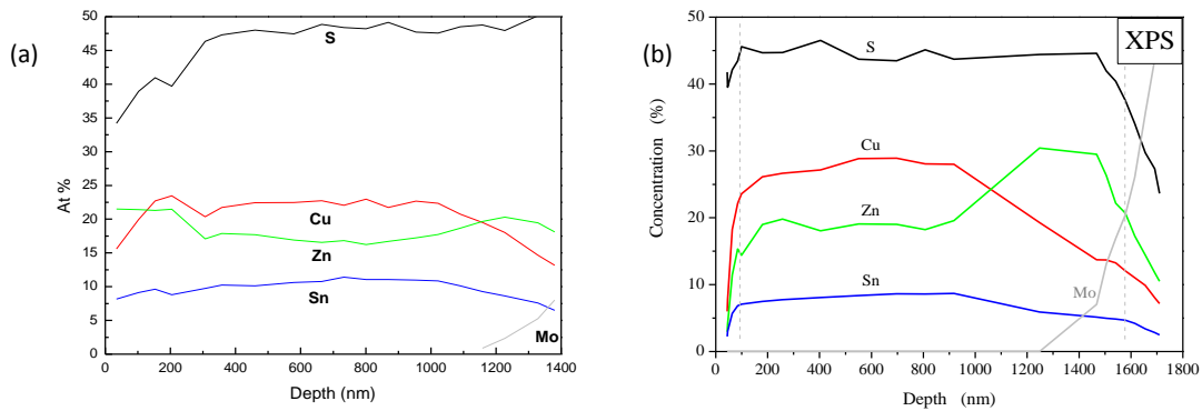
Figura 166. Profili di composizione da misure XPS di un campione di CZTS ottenuto da un precursore co-sputterato (a) e da un precursore stacked evaporato (b)
