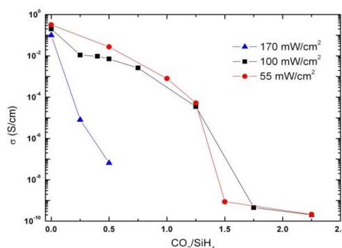
Figura 126. Conduttività elettrica in funzione del rapporto \text{CO}_2/\text{SiH}_4 per le tre serie di campioni
