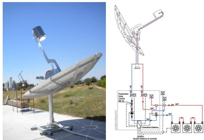
Figura 463. Sistema in prova e lay-out dell'impianto utilizzato per le prove
