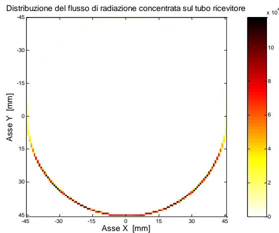
Figura 448. Caso concentratore parabolico lineare: distribuzione della radiazione solare concentrata lungo la circonferenza del tubo ricevitore (valori espressi in \text{W/m}^2 )
