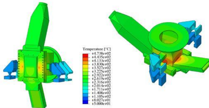
Figura 352. Distribuzione di temperatura nel TA
