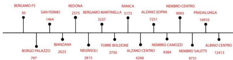
Figura 59. Posizioni [m] delle stazioni della linea tranviaria
