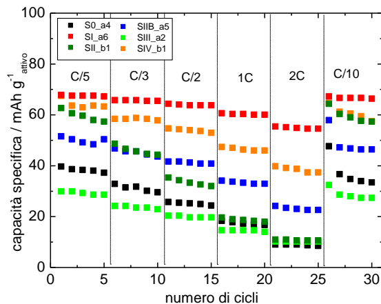
Figura 2. Confronto a 50°C della capacità specifica di scarica alle alte C-rate durante cicli CC(C/10)/CC(C/10) fra 2,5 e 4,5 V degli elettrodi in studio
