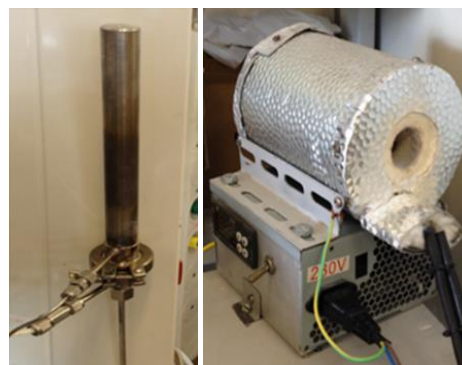
Figura 110. Reattore catalitico e forno di riscaldamento
