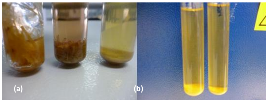
Figura 99. Immagini relative alla degradazione della paglia in tubi Hungate: nella foto a sinistra la paglia nel tempo iniziale, intermedio, e finale delle prove; nella foto a destra ciò che resta della paglia inizialmente fornita come substrato ai due ceppi fungini
