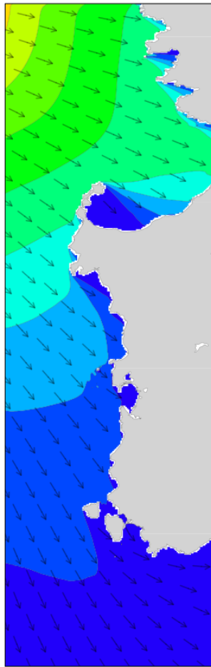
Figura 213. Esempio di previsione del valore dell'energia e della direzione per la costa occidentale della Sardegna, Golfo di Napoli, e Lampedusa
