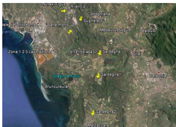
Figura 308. Dislocazione delle sei stazioni di monitoraggio all'interno della concessione mineraria "Monte Sinni" della Carbosulcis S.p.A.
