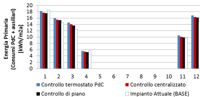
Figura 424. Energia primaria richiesta, al variare della tipologia impiantistica, per la climatizzazione invernale di una superficie unitaria dell'edificio
