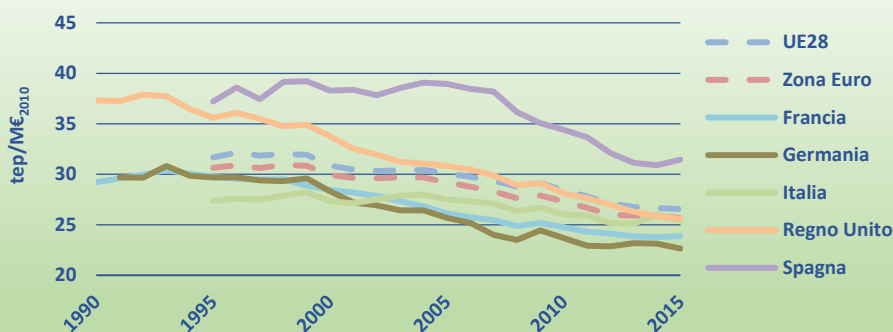
Figura 2.25 – Intensità energetica del settore trasporti in alcuni paesi europei (tep/M€ 2010 ), anni 1990-2015
