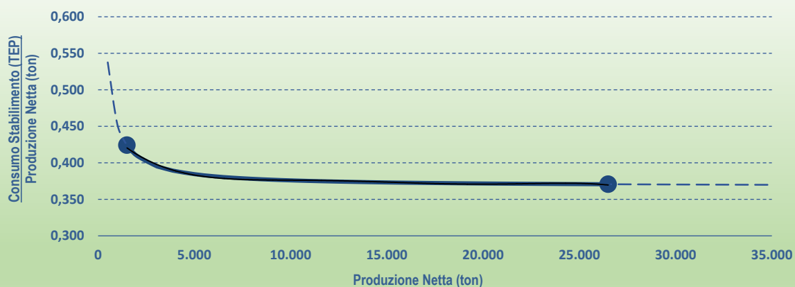
Figura 4.5 – Indice di prestazione energetica generale per lo stabilimento di una fonderia di ghisa
