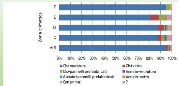
Figura 5.3 - Edifici scolastici. Tipologie costruttive per zone climatiche
