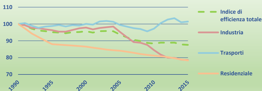
Figura 2.26 – Indice di efficienza energetica ODEX (1990=100), anni 1990-2015
