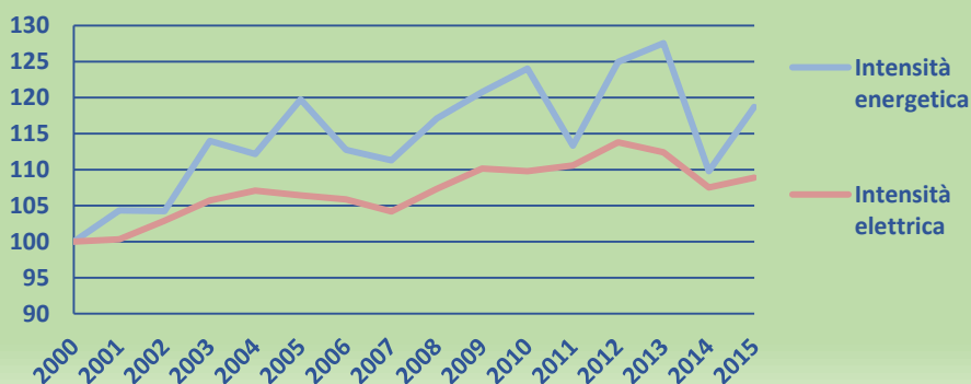
Figura 2.23 – Intensità energetica finale ed intensità elettrica nel residenziale (2000=100), anni 2000-2015
