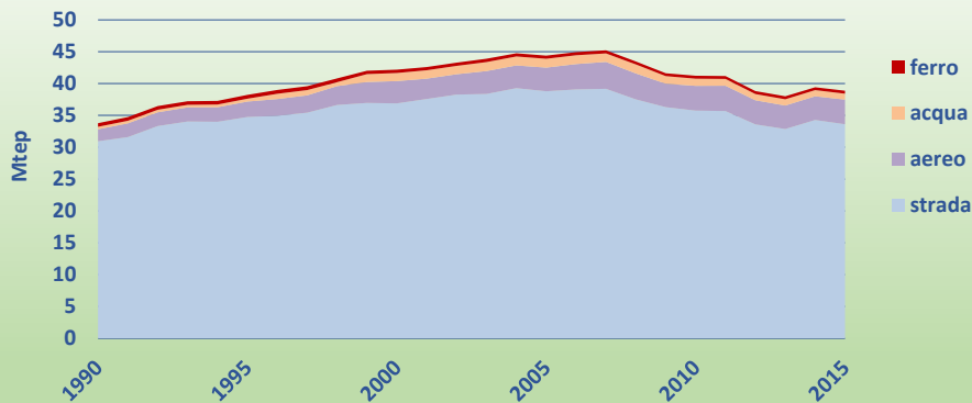
Figura 2.17 – Consumi finali nei trasporti per modalità (Mtep), anni 1990-2014
