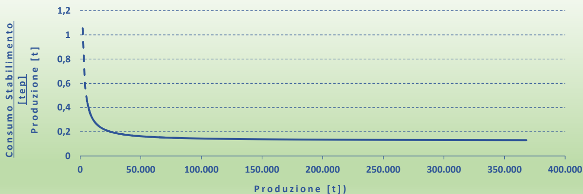
Figura 4.7 – Indice di prestazione generale di stabilimento per la produzione di tissue
