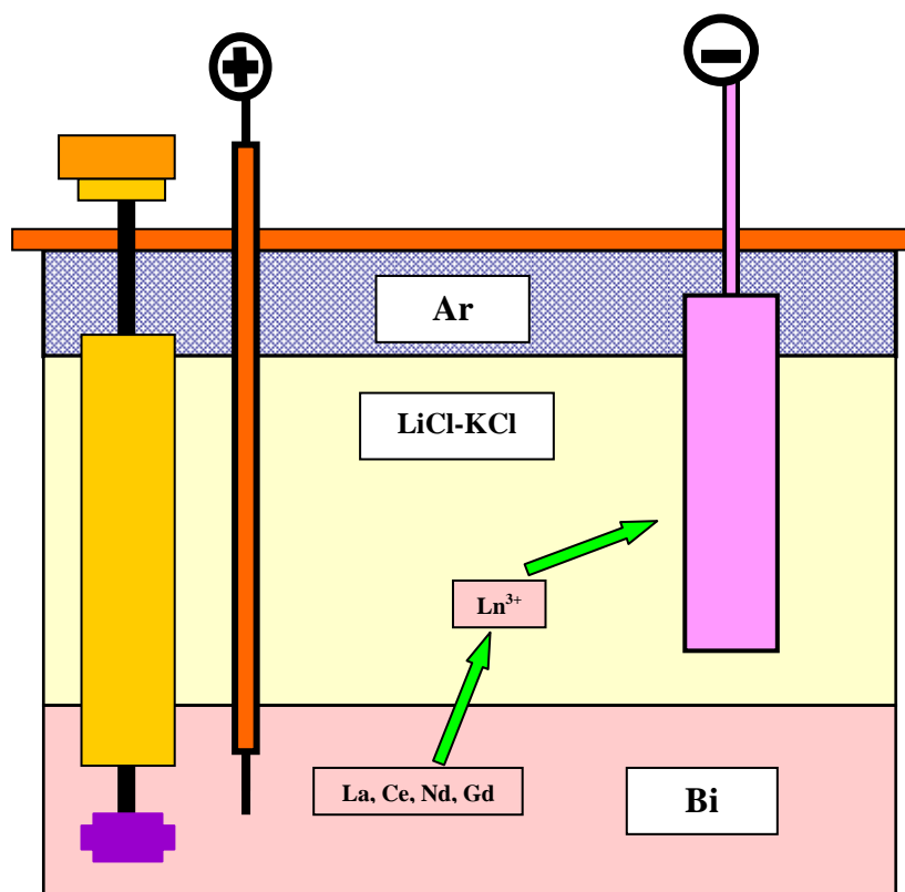
Figura 5 – Schema del processo di elettrolisi per la rimozione di metalli inquinanti dal bismuto fuso
