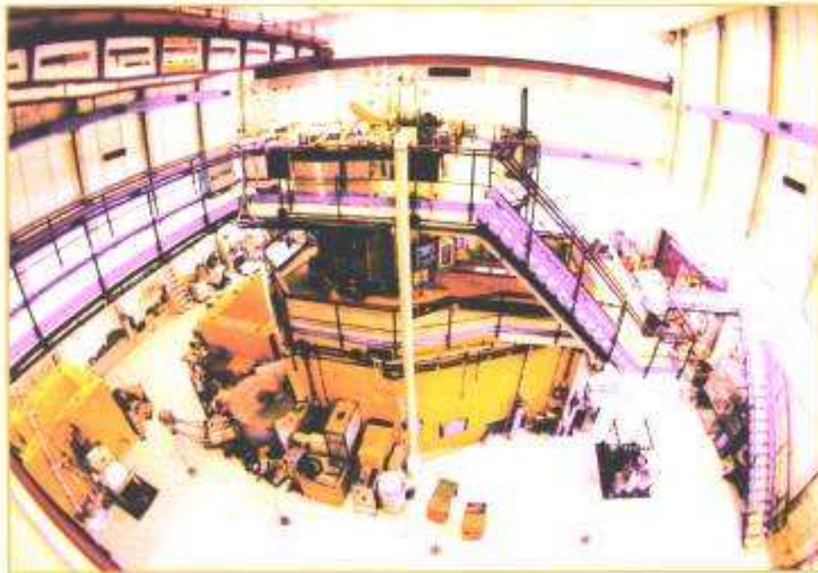
Fig. 3-36 Vista della hall tecnologica del reattore TRIGA RC-1 dell'ENEA
