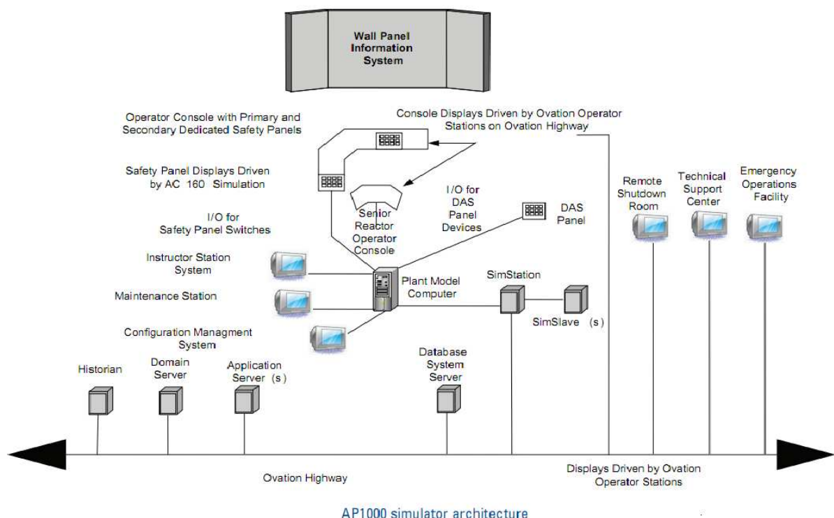
Fig. 5-2 Architettura hardware di un simulatore full scale dell'impianto AP1000 (Westinghouse)
