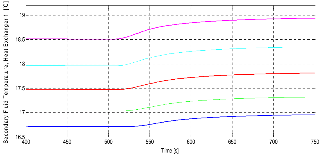
Fig. 3-34 Distribuzione assiale del campo di temperature nel fluido secondario all'interno del mantello dello scambiatore 1
