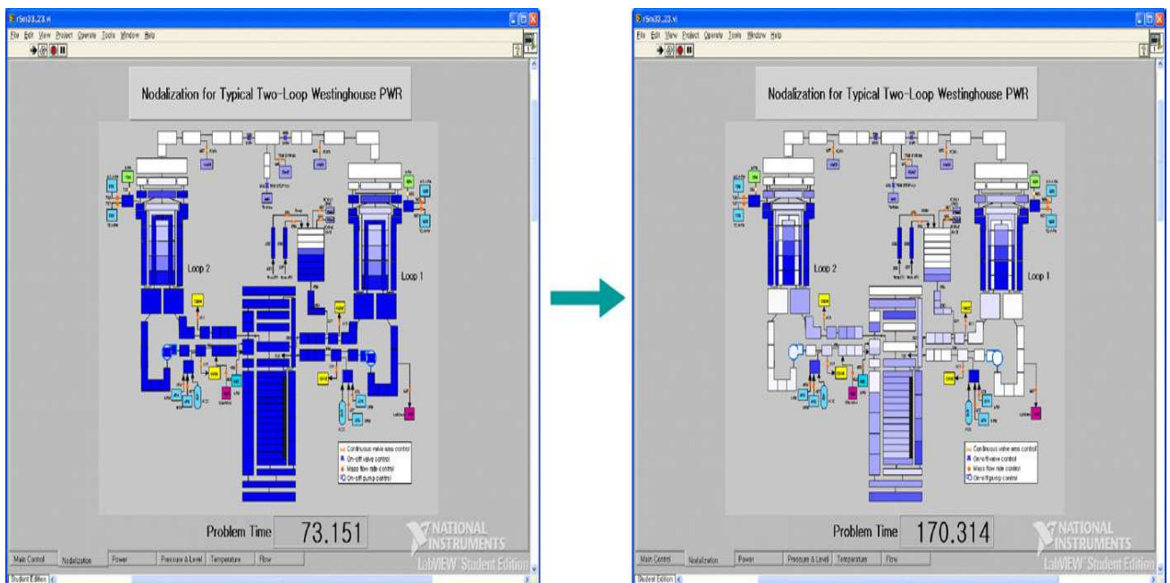
Fig. 3-52 Nodalizzazione primario
