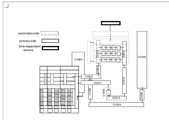
Figura 15. – Nodalizzazione VVER-1000 Generico – Melcor RCS
