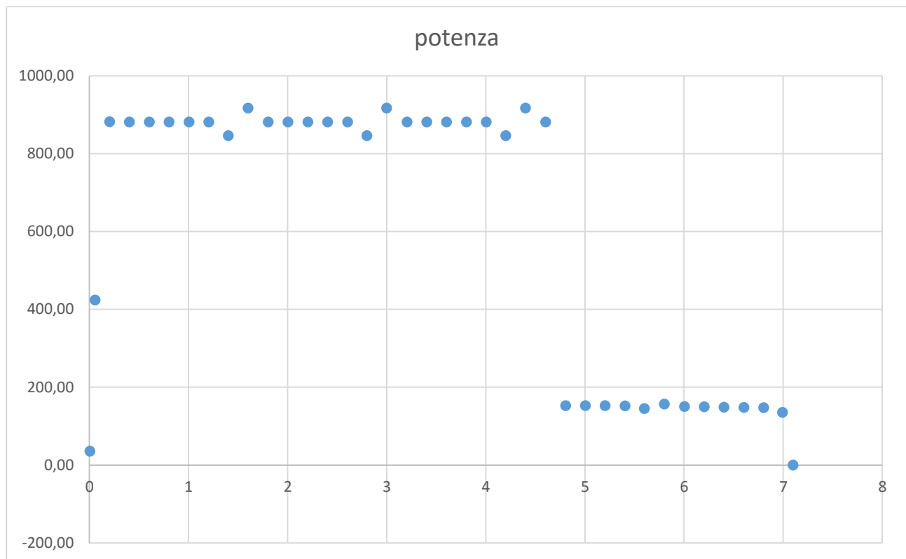
Figura 19. Distribuzione di potenza ottenuta dall'integrazione del profilo reale
