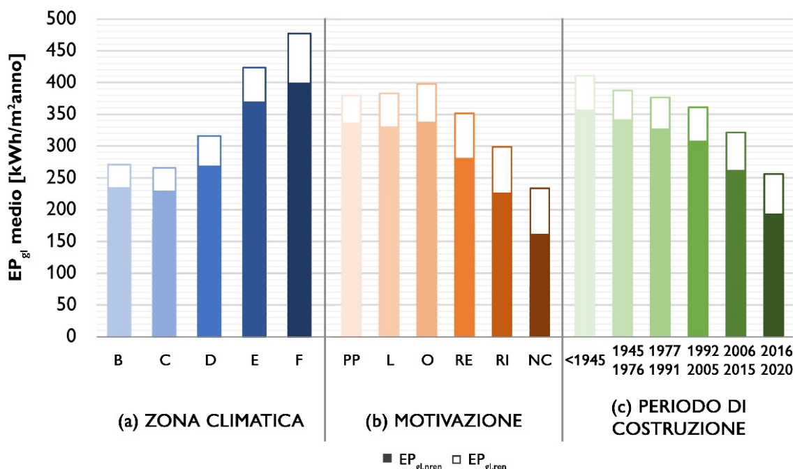
Figura 2. Distribuzione dell' EP_{gl} medio per zona climatica (a), motivazione (b) e periodo di costruzione (c) per gli immobili non residenziali. PP: passaggio di proprietà; L: locazione; A: altro; RE: riqualificazioni energetiche; RI: ristrutturazione importante; NC: nuove costruzioni (fonti: Regioni e Province Autonome e SIAPE)
